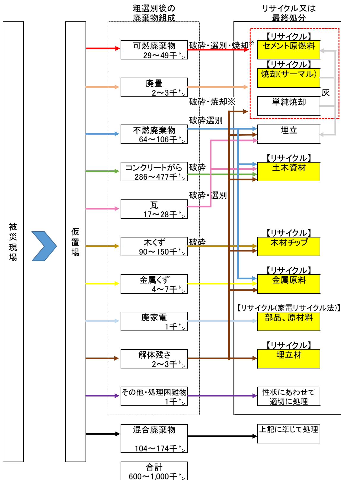
図3-1 処理フロー
