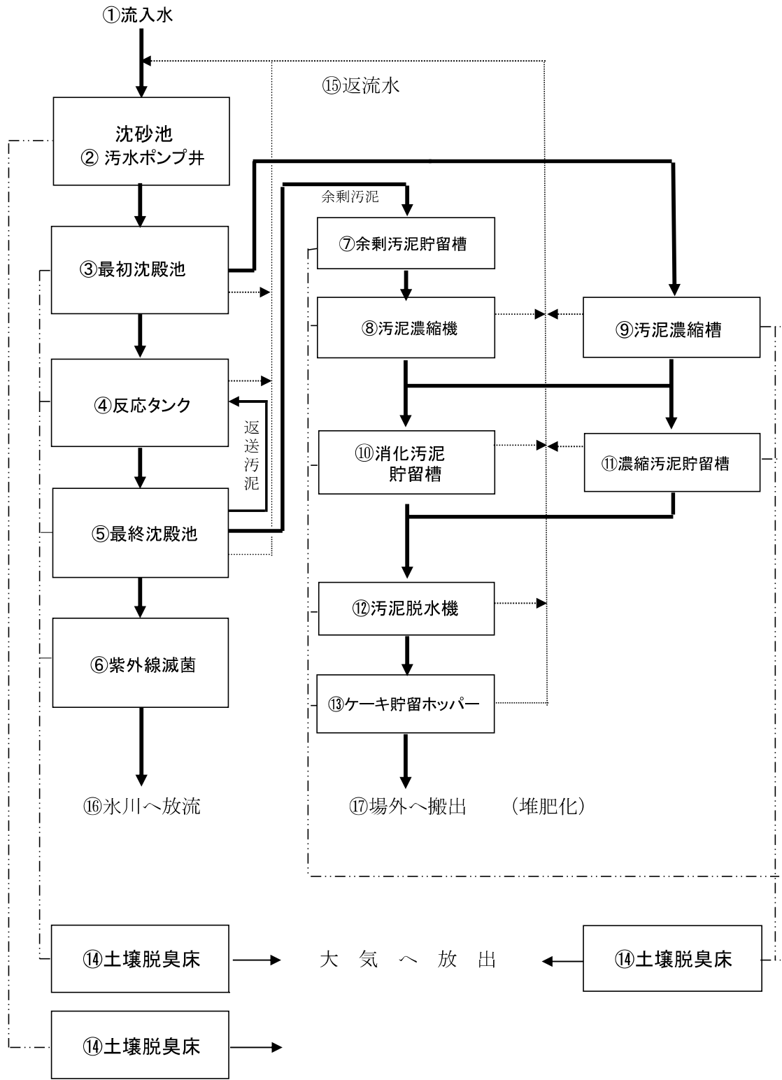
(別添1ー5)八代北部浄化センターフローシート
