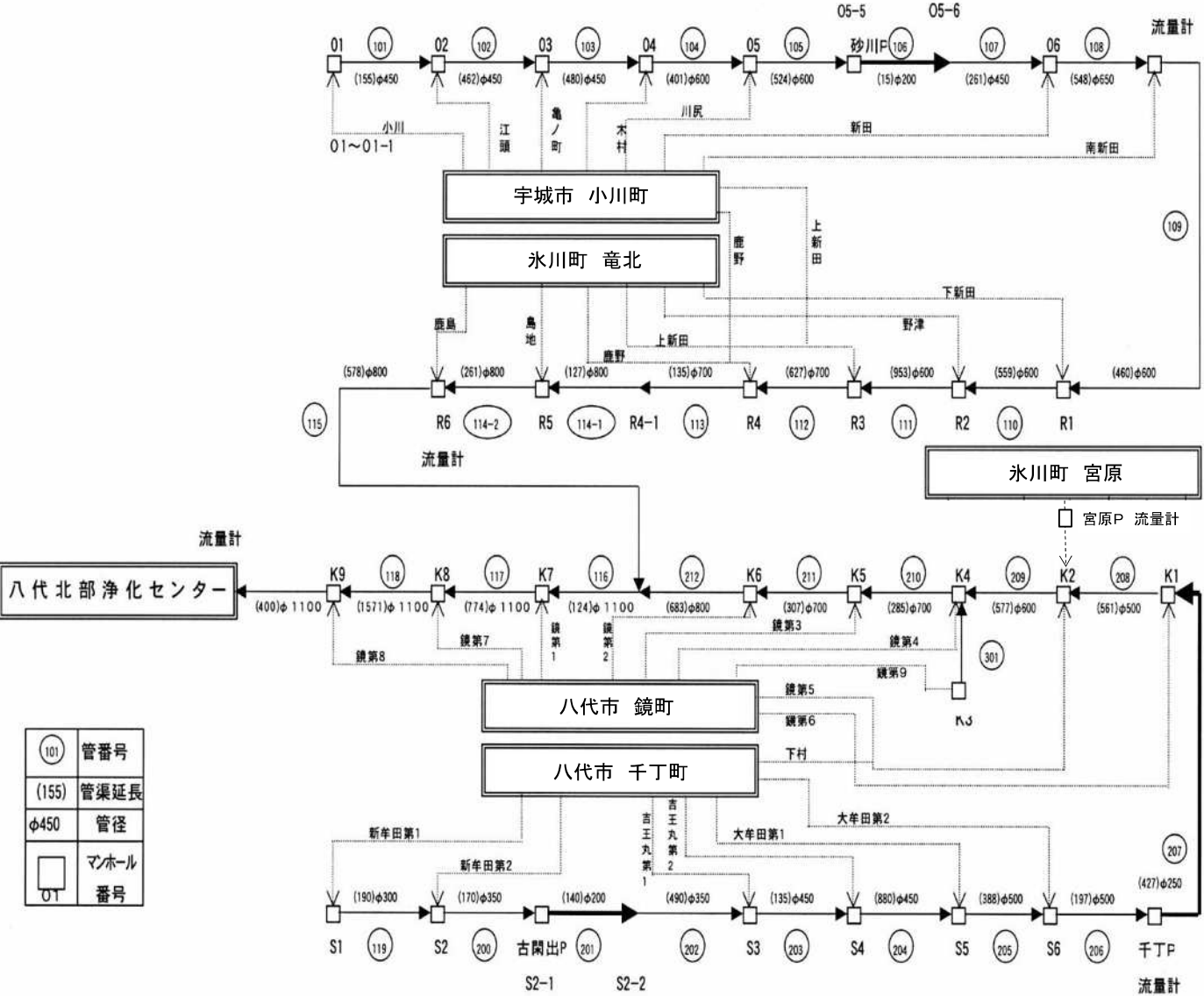
(別添1-6)八代北部流域下水道 幹線図
