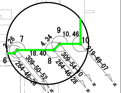
拡大図 S=1:1,000
