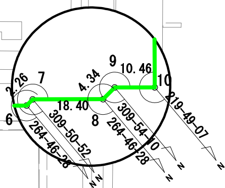
拡大図 S=1:1,000
