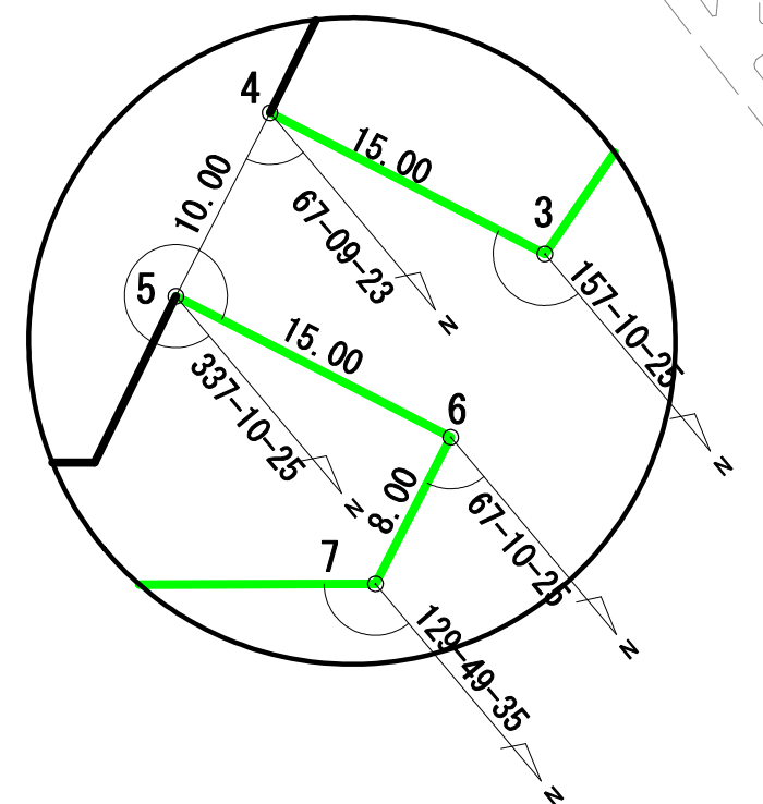
拡大図 S=1 : 500
