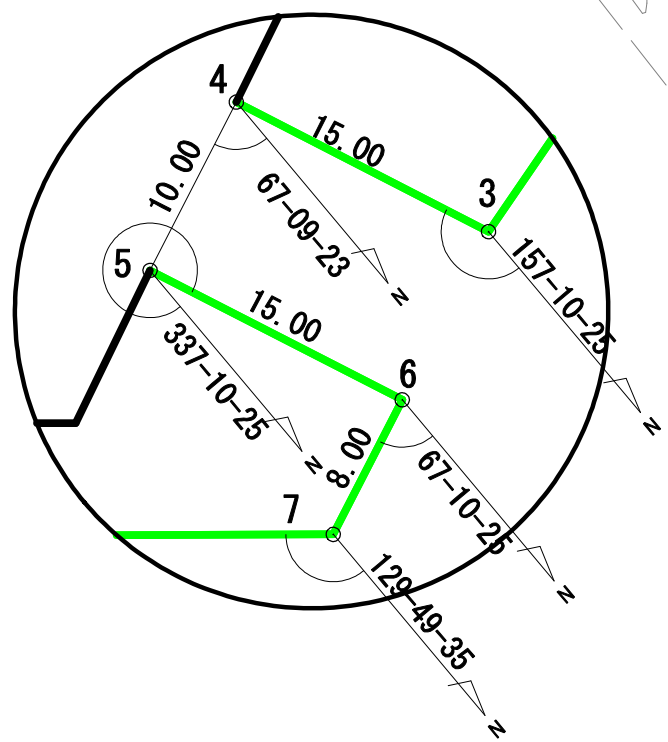
拡大図 S=1:500
