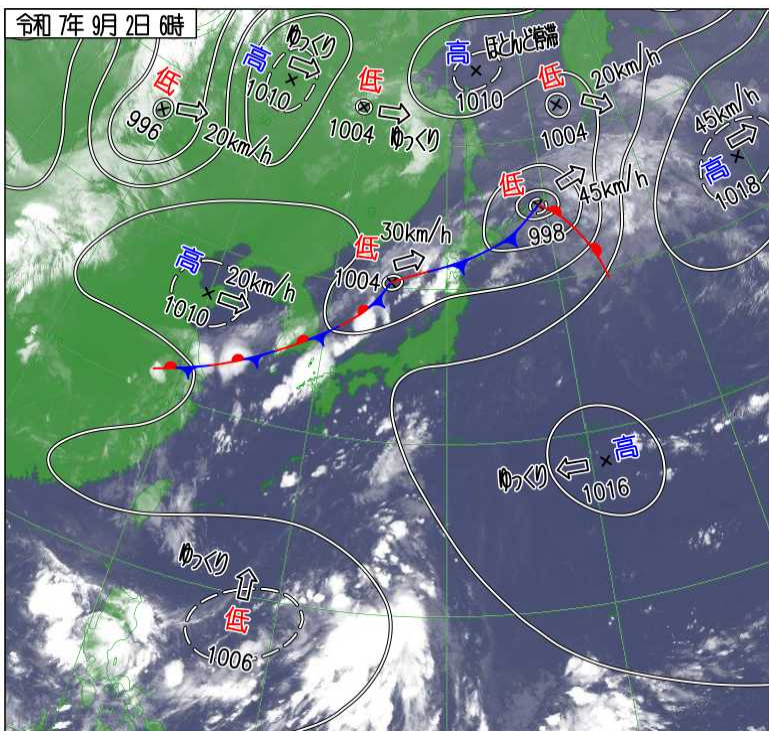
地上天気図（2日6時）
