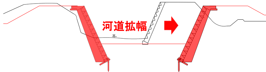
千間江湖 河道拡幅
