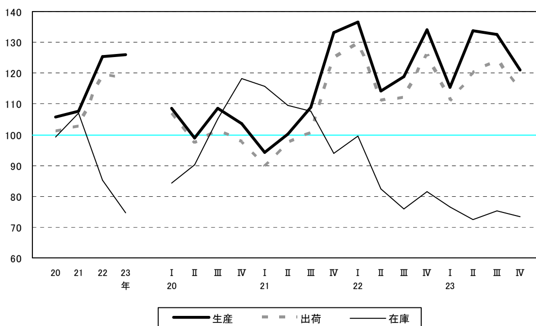
第12図 化学工業の推移(H17=100)
