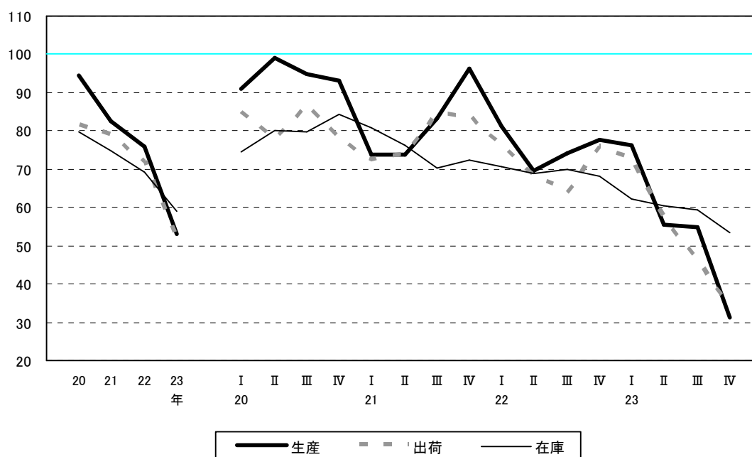
第20図 鉱業の推移(H17=100)
