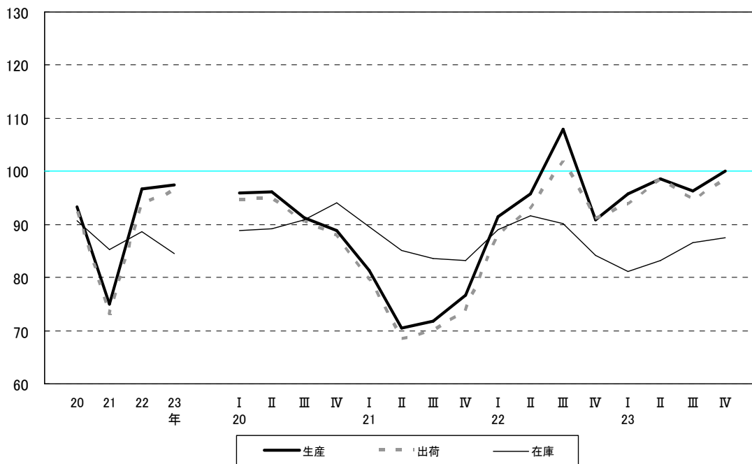
第21図 最終需要財の推移(H17=100)
