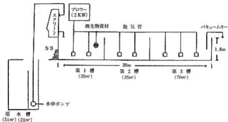
第1図 処理施設のフローシート
