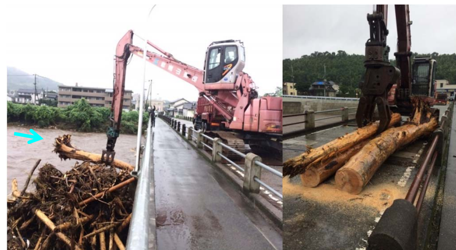
平成28年6月25日 つかみ具付き建設機械による撤去作業
