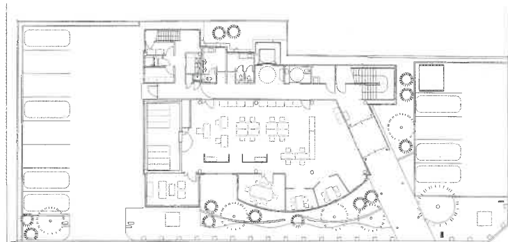
1階平面図
