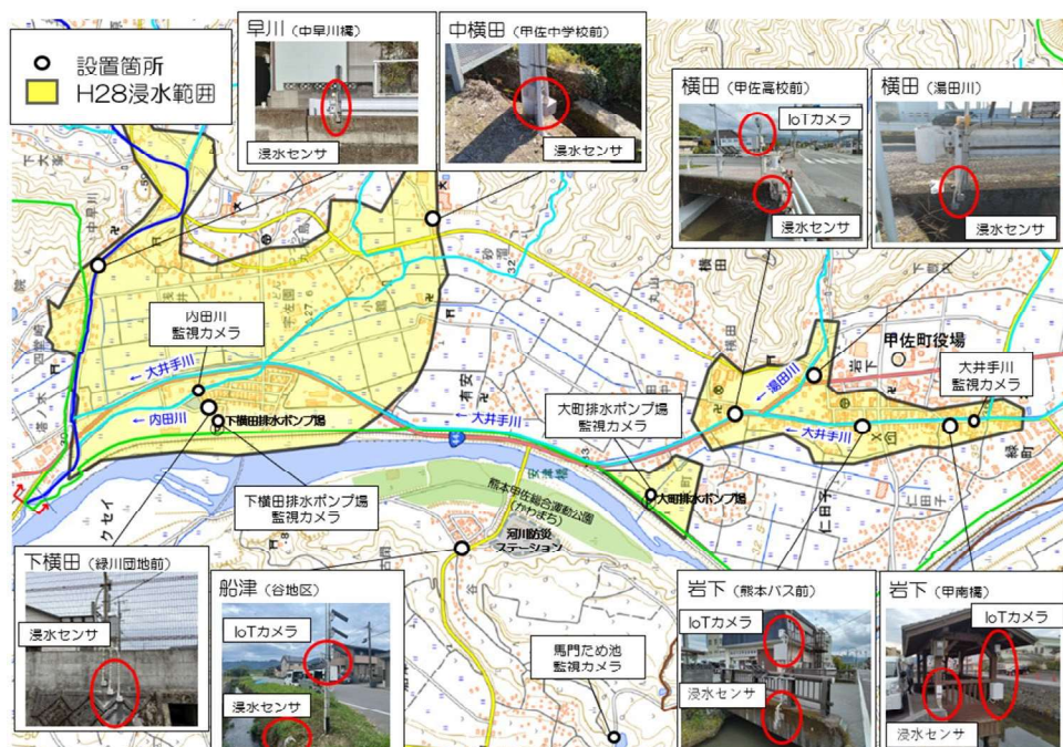
図 12-7 甲佐町 浸水センサ設置状況
