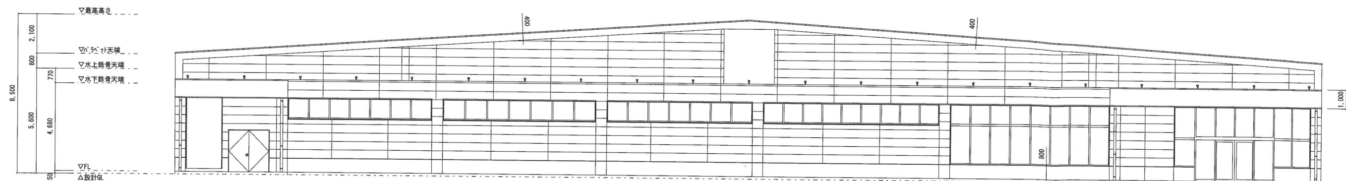
南東側立面図
