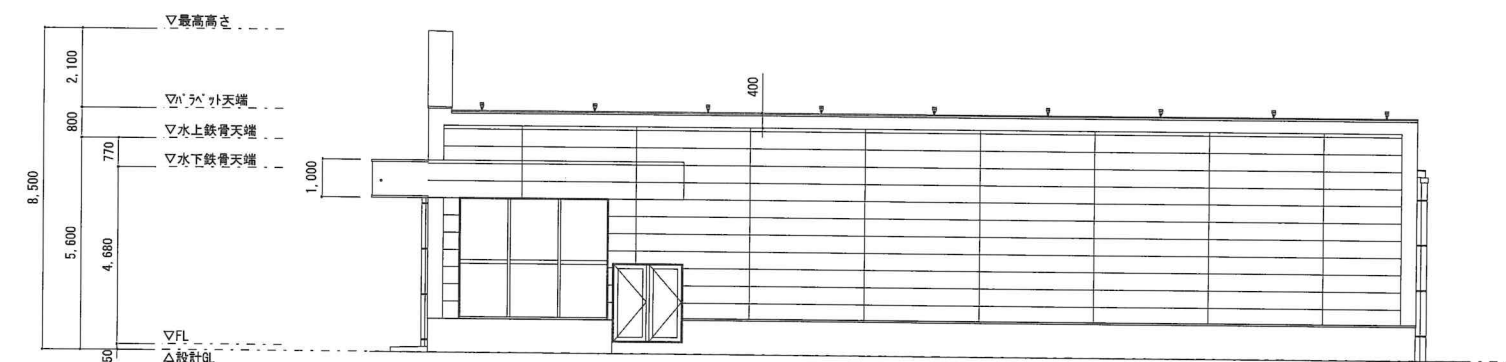
北東側立面図
