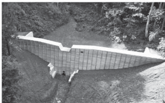
溪間工（谷止工）
