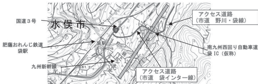
南九州西回り自動車道芦北出水道路の整備状況（袋IC付近）
