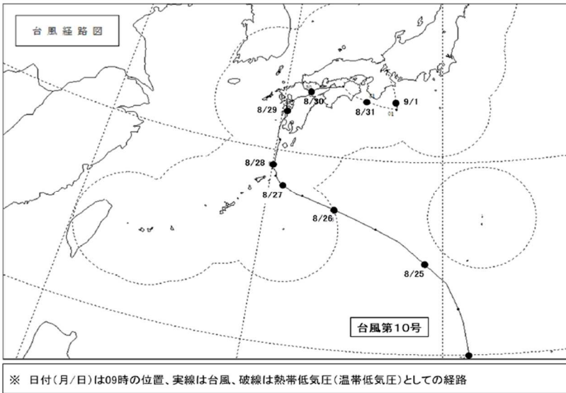
（４）２０２２年（令和４年）に九州に上陸した台風の経路図
