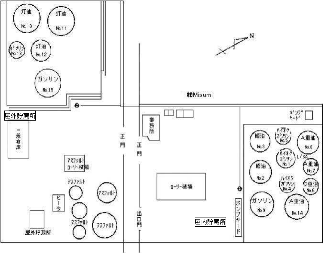
図4 出光ターミナルネットワーク(株)八代油槽所配置図
