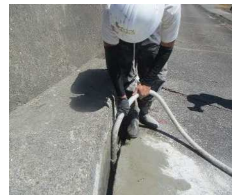
波返工空洞箇所へのグラウト注入（八代市）
