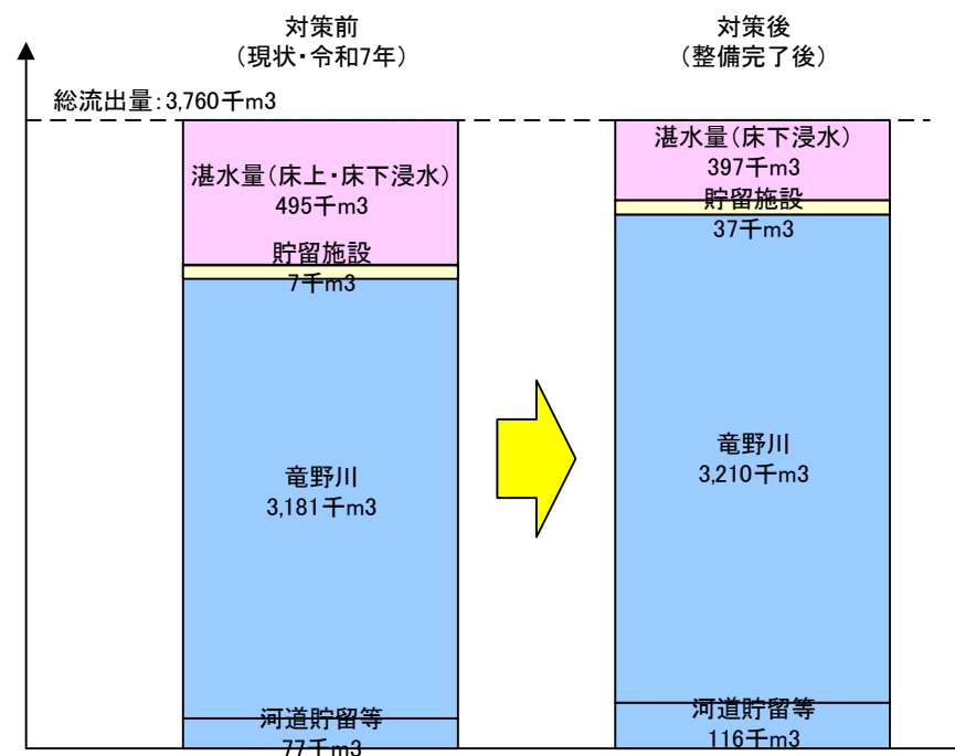
本計画における対策効果（湛水量の減少）
