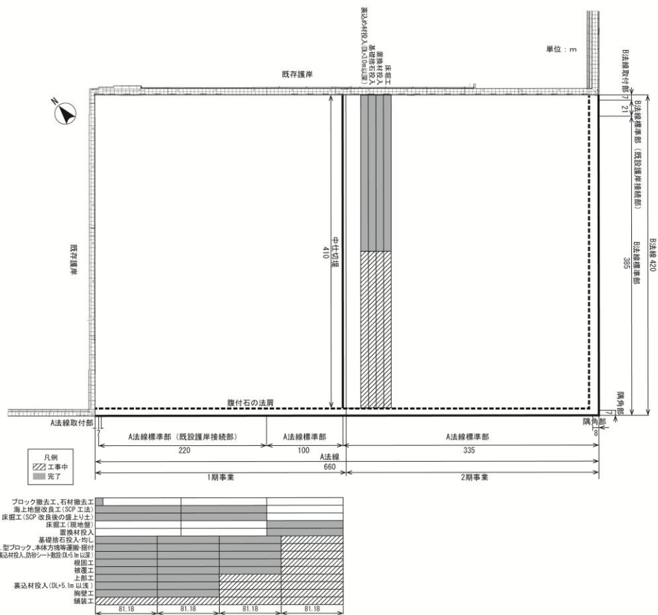
図 2-19(2) 護岸工の工事進捗図 (1 期)
