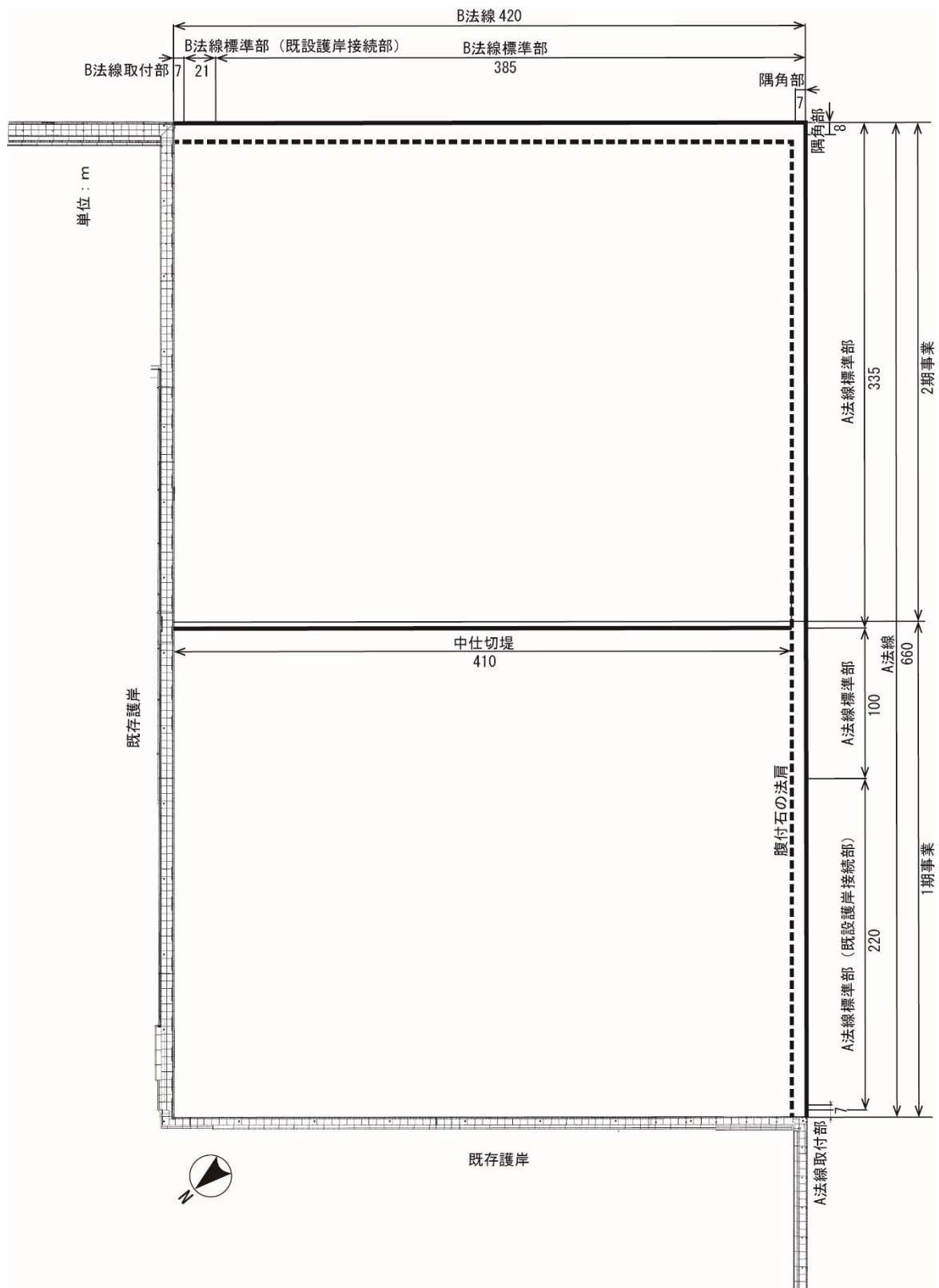
図 2-4 護岸配置図
