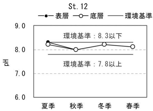
圖 7.5-4(1) 現地調查結果 (pH)
