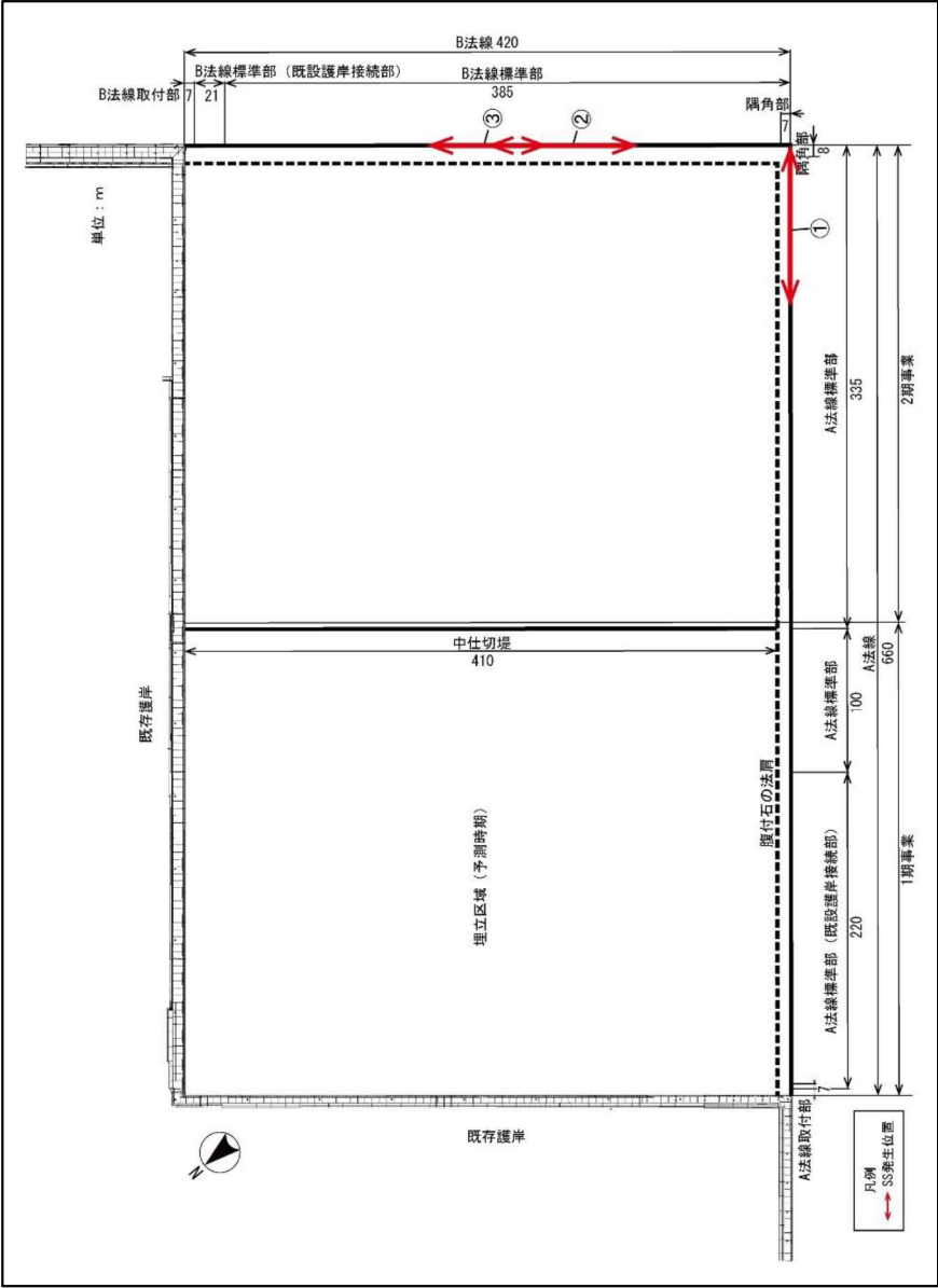
図 7.5-16 SS 発生位置図
