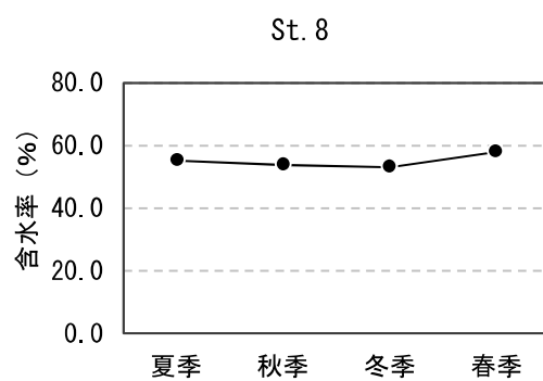
図 7.5-9(9) 現地調査結果 (含水率)
