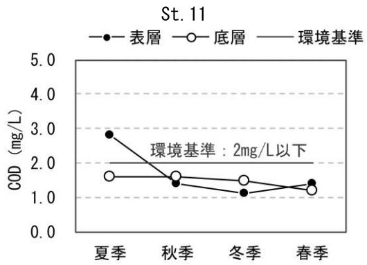
図 7.5-4(3) 現地調査結果 (COD)
