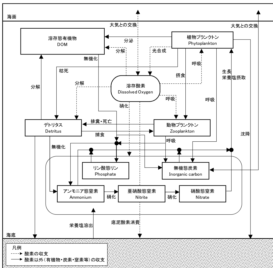
図 7.5-19 水質モデルの概念図
