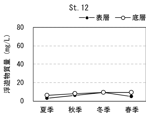
図 7.5-4(7) 現地調査結果 (浮遊物質量)
