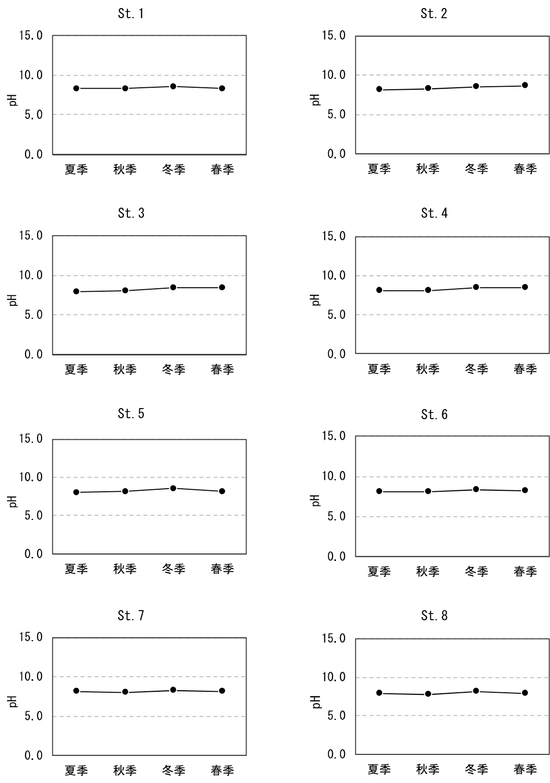
図 7.5-9 (7) 現地調査結果 (pH)
