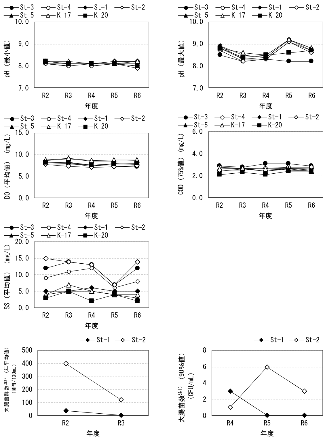
図 7.5-3 生活環境項目の経年変化
