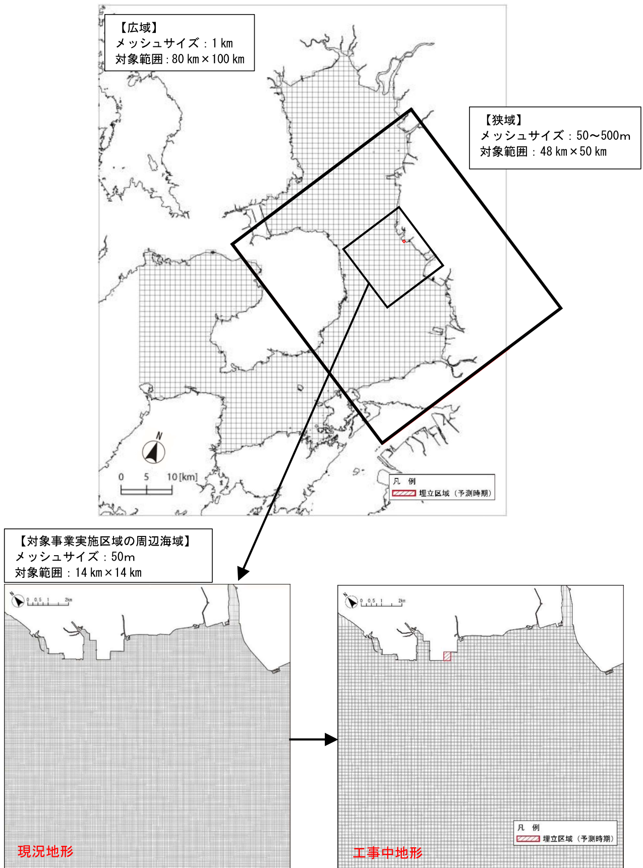
図 7.5-13 格子分割図
