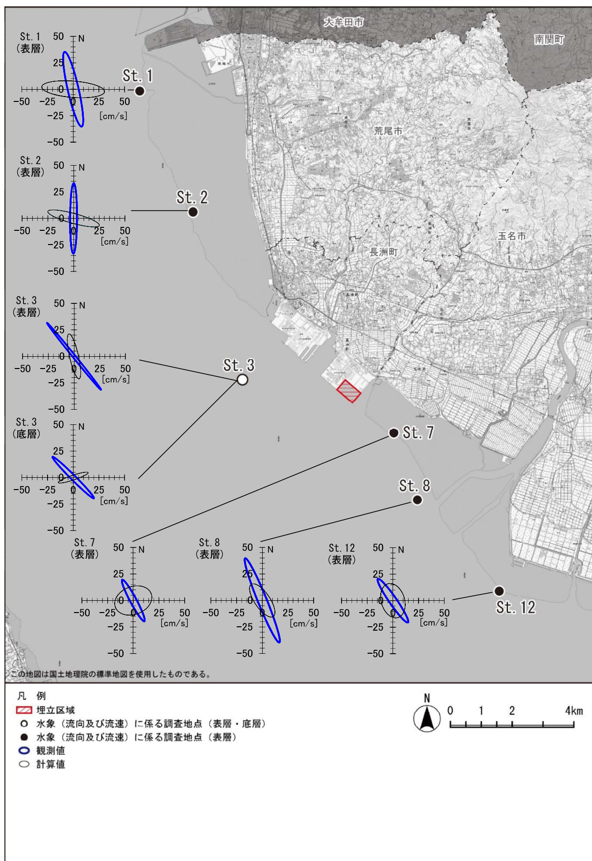
図 7.4-23(2) 調査地点における M_2 分潮の潮流楕円の観測値と計算値との比較（夏季） 注 1) 表層 観測値：海面下 0.5m、計算値：第 1 層（0～3m） 底層 観測値：海底上 1.0m、計算値：海底直上層
