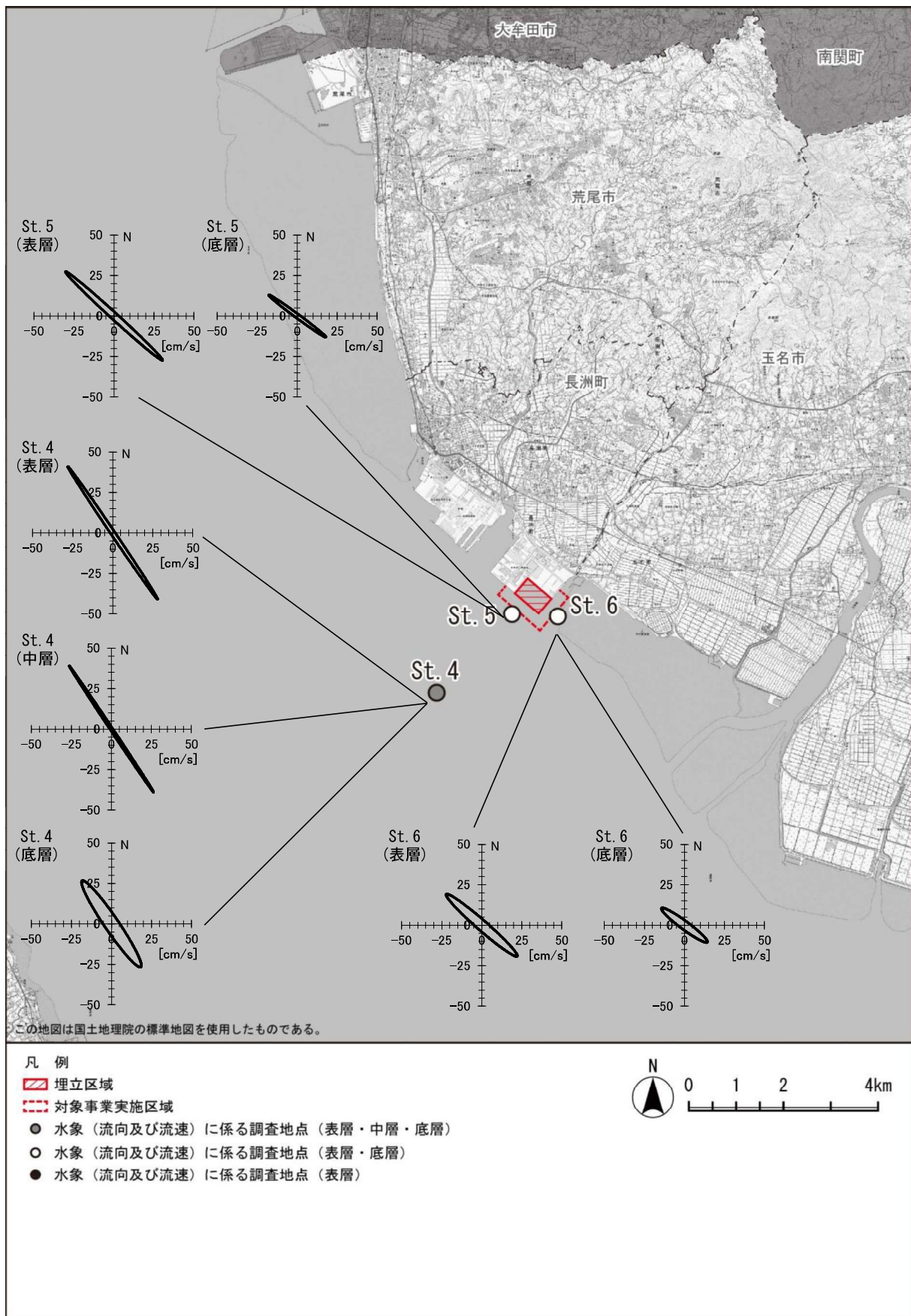
図 7.4-8(1) 潮流橢円図 ( M_2 分潮) (夏季)
