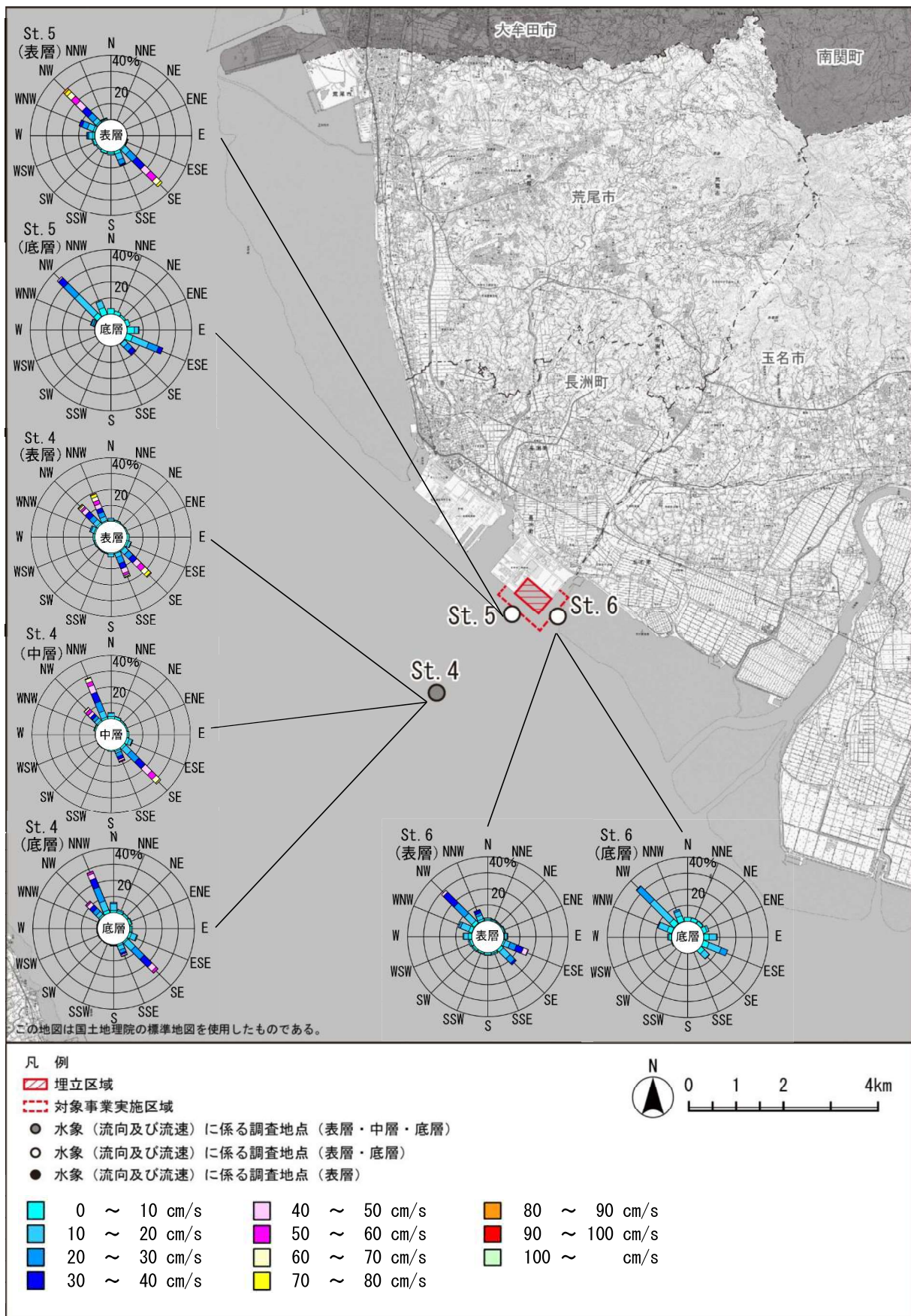
図 7.4-7(1) 流向・流速頻度分布図（冬季）
