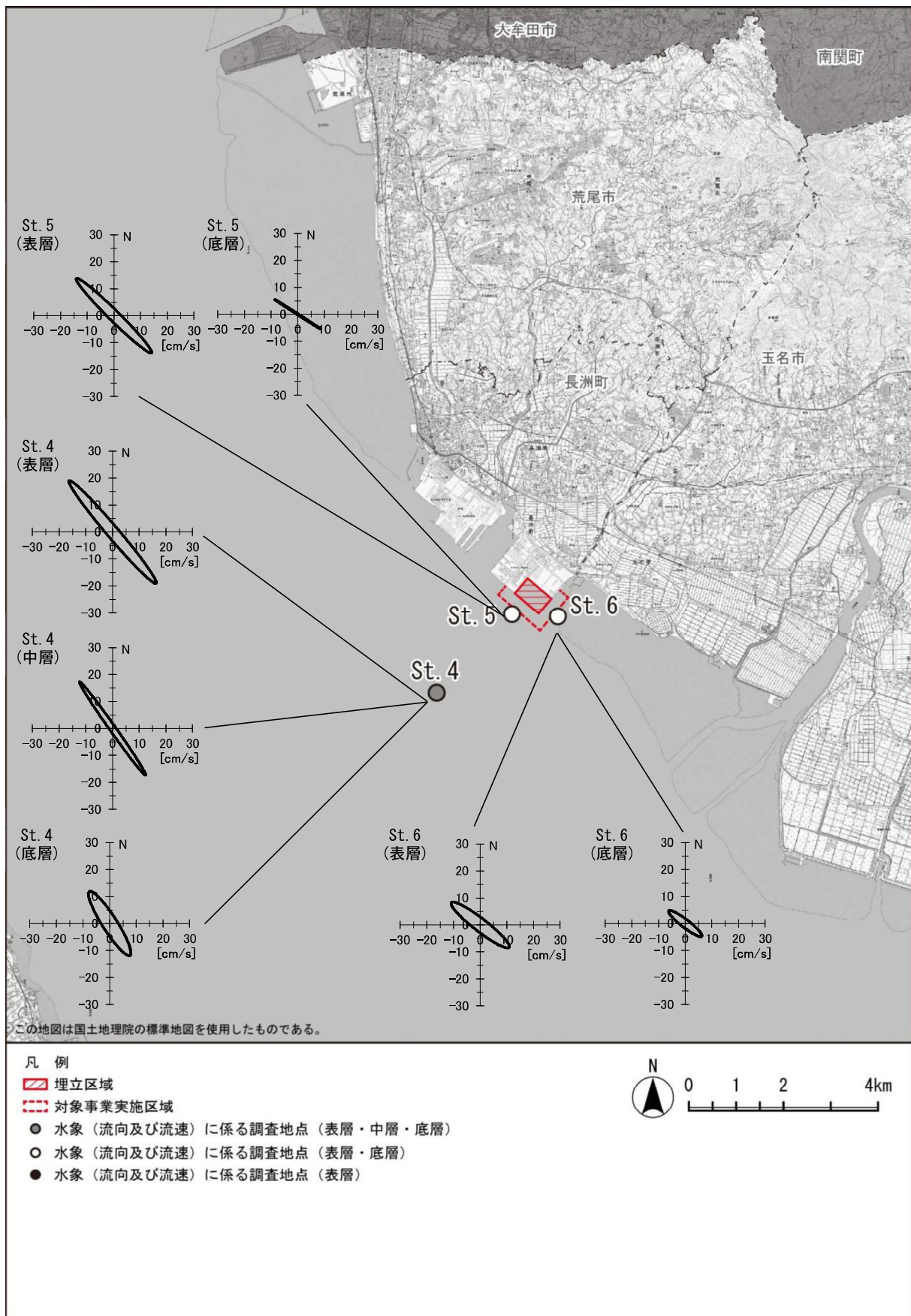
図 7.4-10(1) 潮流楕円図 ( S_2 分潮) (夏季)
