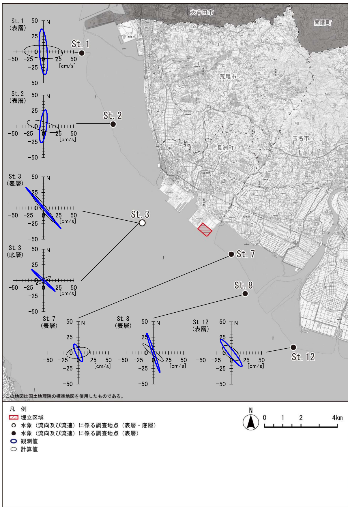
図 7.4-24(2) 調査地点における M_2 分潮の潮流楕円の観測値と計算値との比較（冬季）
