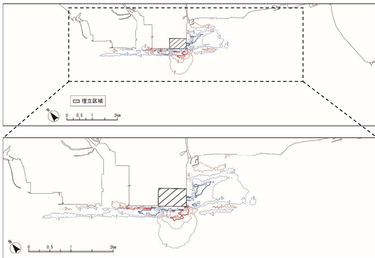
図 7.4-28 (2) 流速差図 (事業ありー事業なし: 冬季上げ潮最強時 ( M_2+S_2 分潮))
