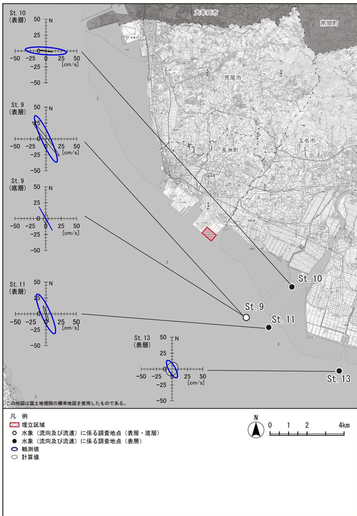
図 7.4-23(3) 調査地点における M_2 分潮の潮流楕円の観測値と計算値との比較（夏季）
