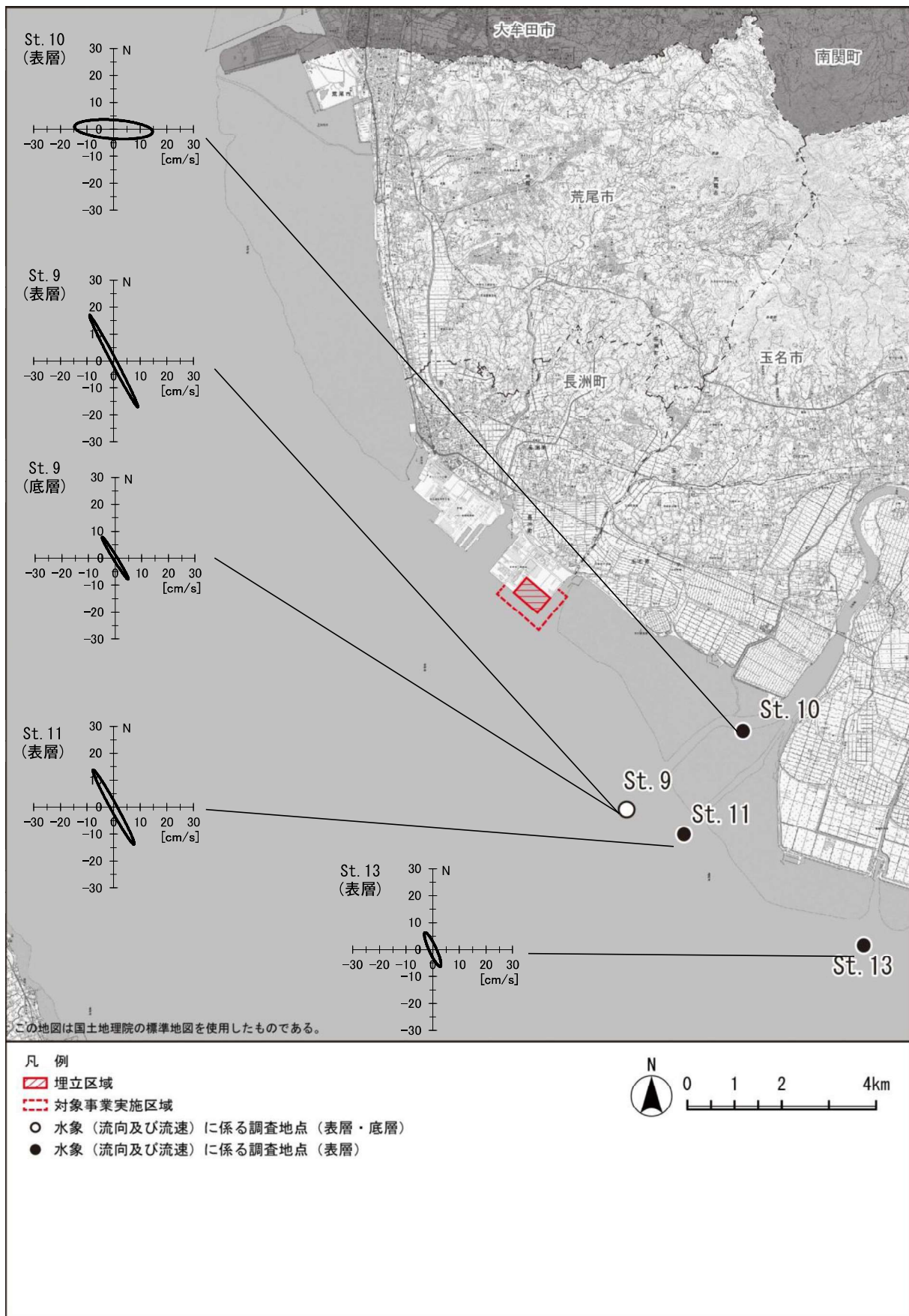
図 7.4-10(3) 潮流橢円図 ( S_2 分潮) (夏季)
