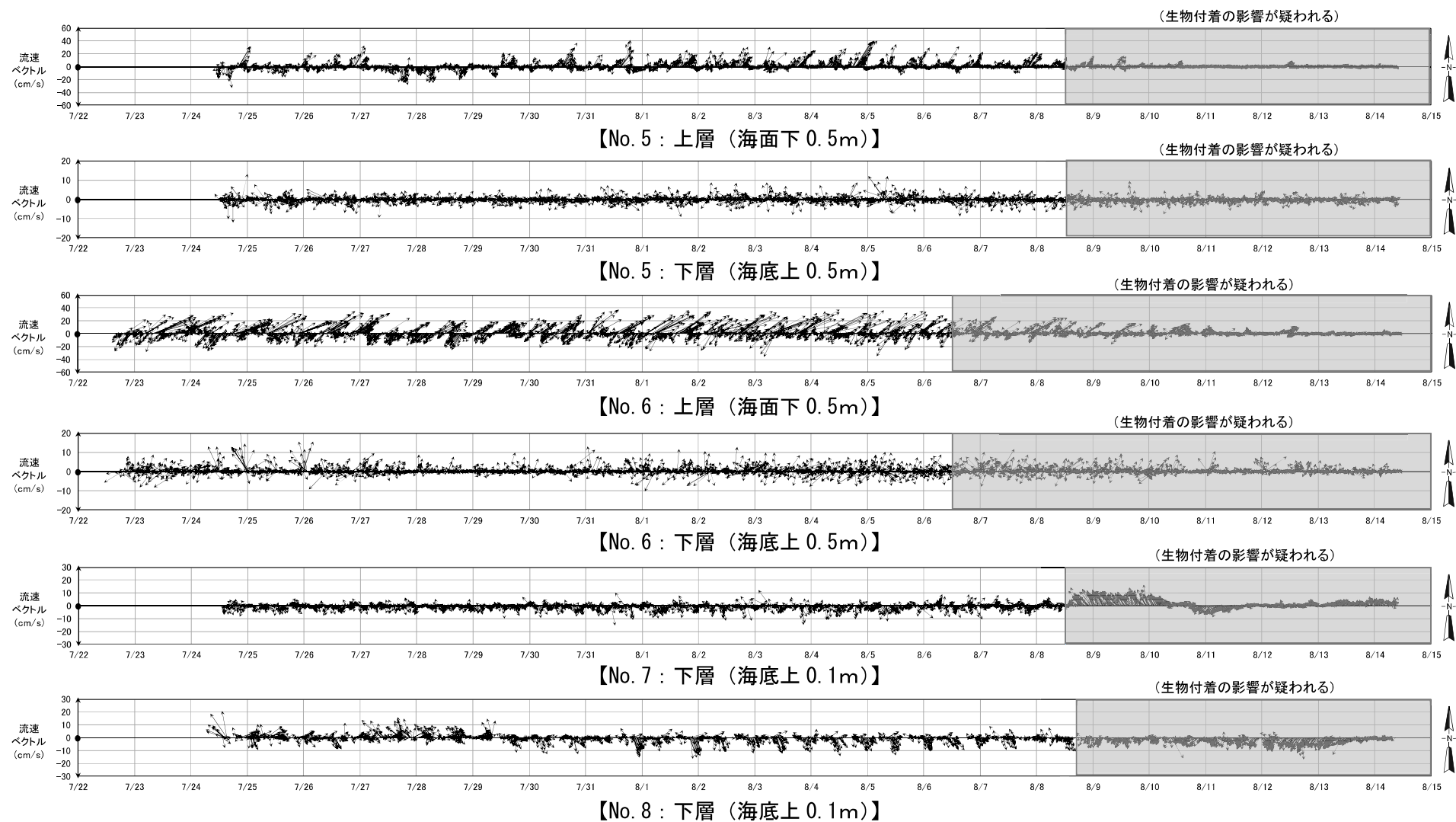
図 7.4-5(1) 潮流の調査結果 (令和 2 年度)
