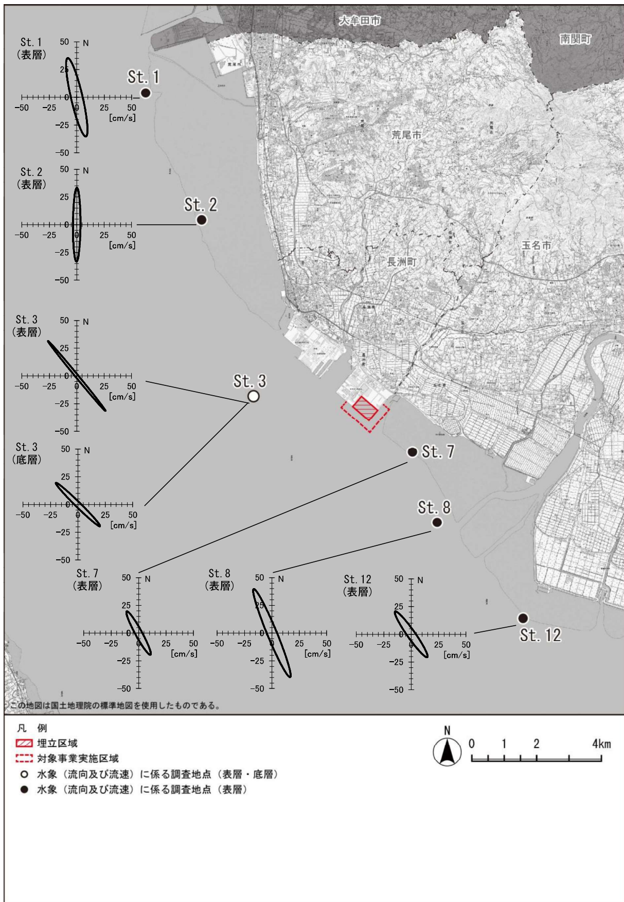
図 7.4-8(2) 潮流橢円図 ( M_2 分潮) (夏季)
