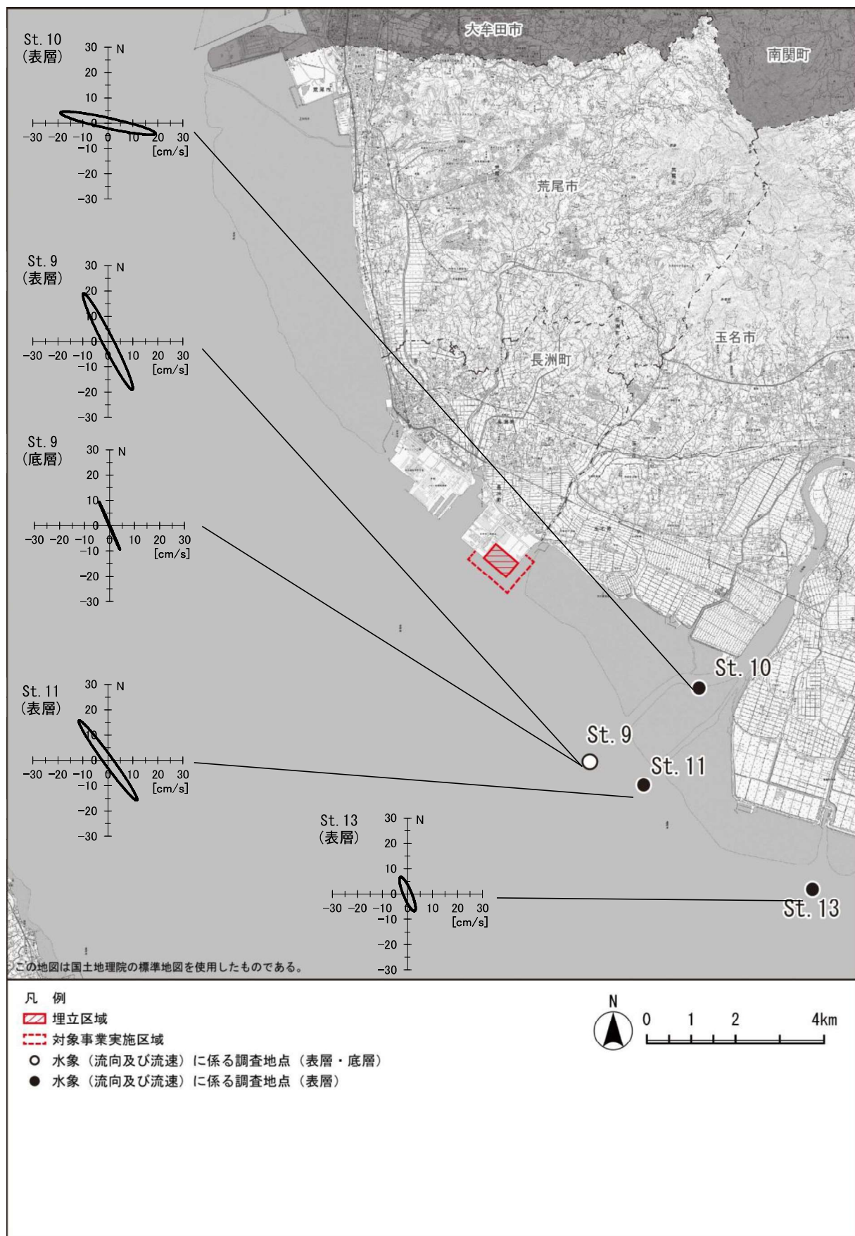
図 7.4-11(3) 潮流橢円図 ( S_2 分潮) (冬季)
