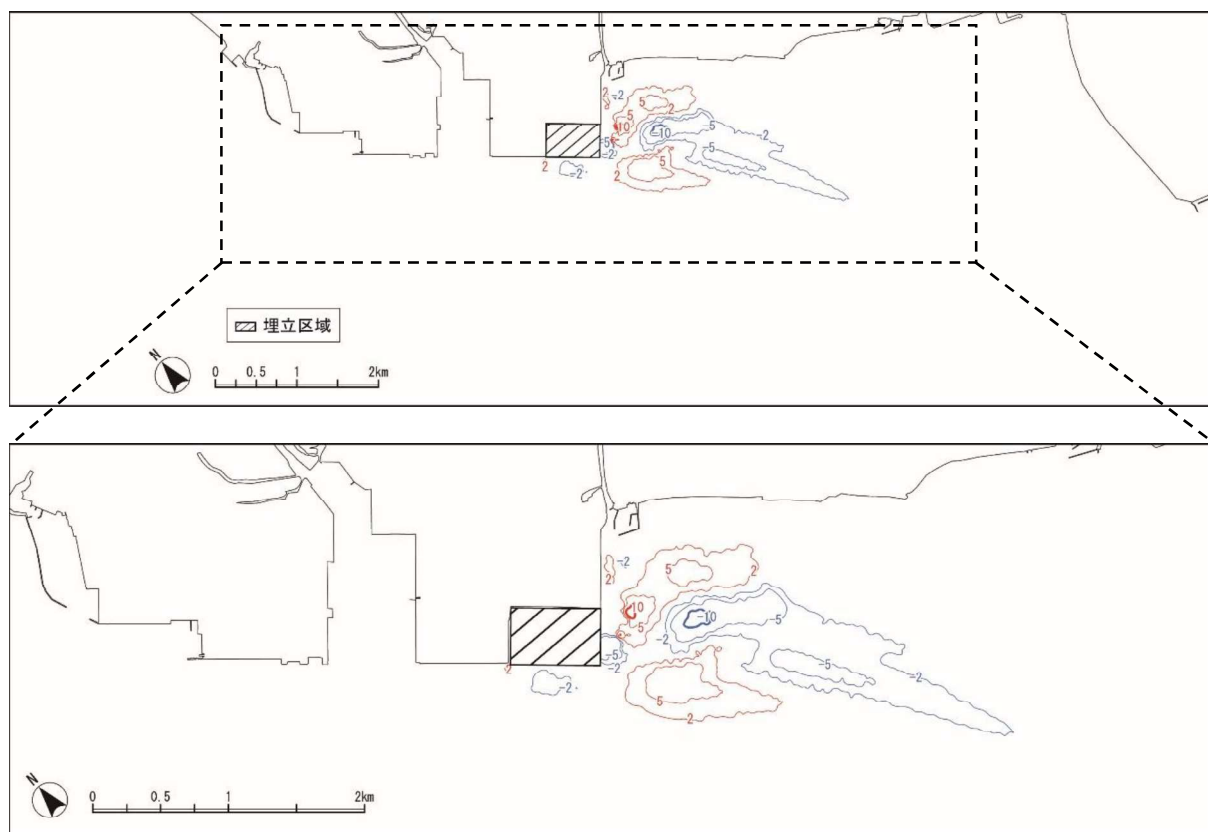
図 7.4-28(4) 流速差図（事業ありー事業なし：冬季下げ潮最強時（ M_2+S_2 分潮））
