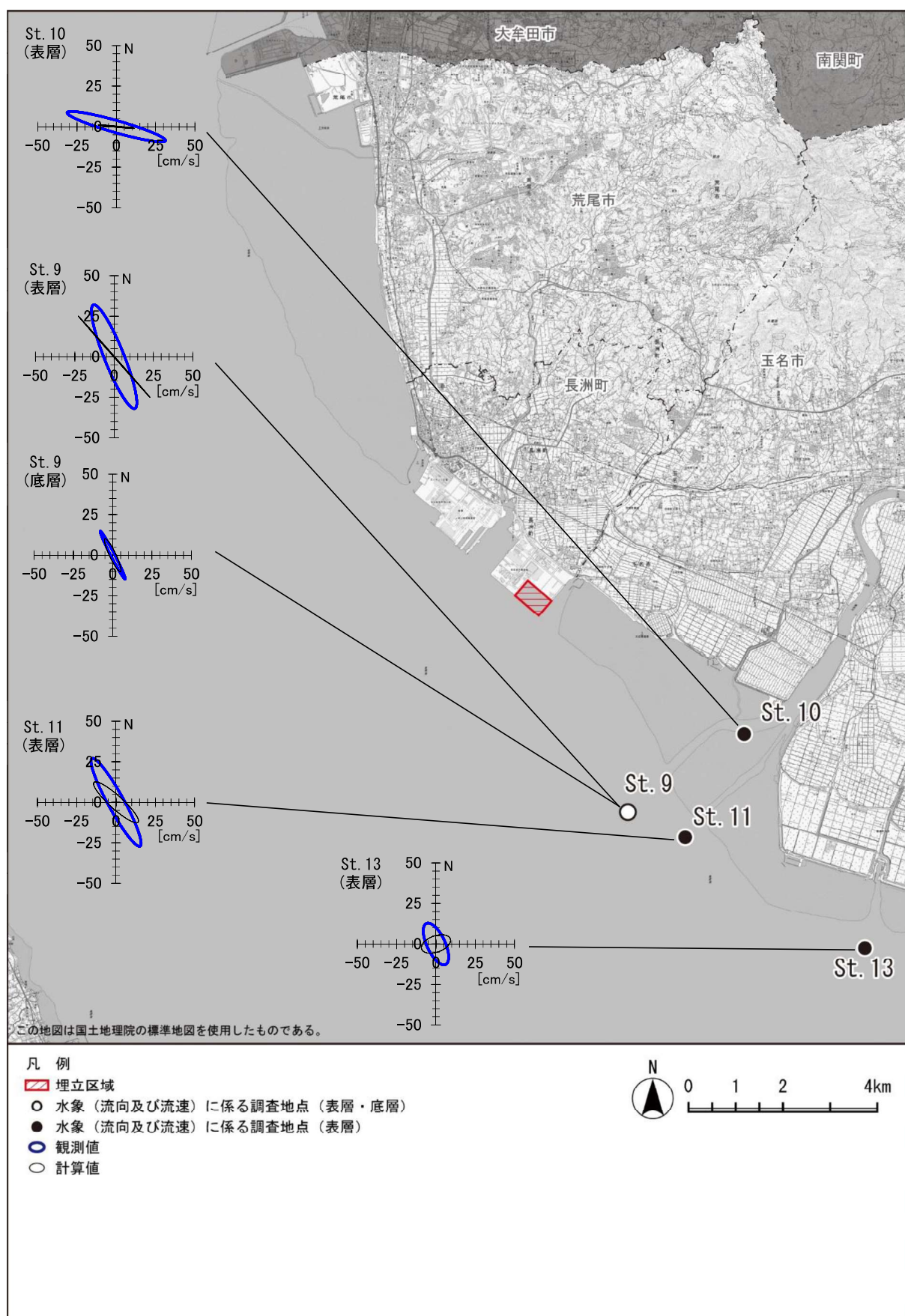
図 7.4-24(3) 調査地点における M_2 分潮の潮流楕円の観測値と計算値との比較（冬季）
