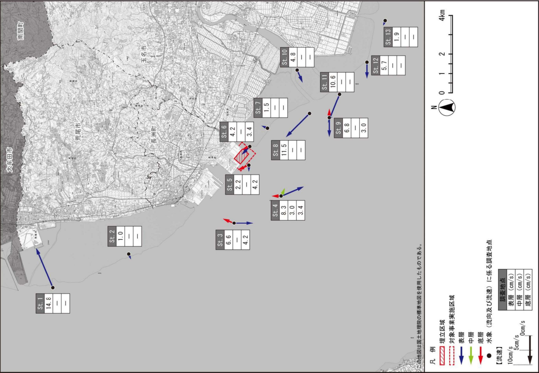
図 7.4-13(1) 恒流の分布図 (夏季)
