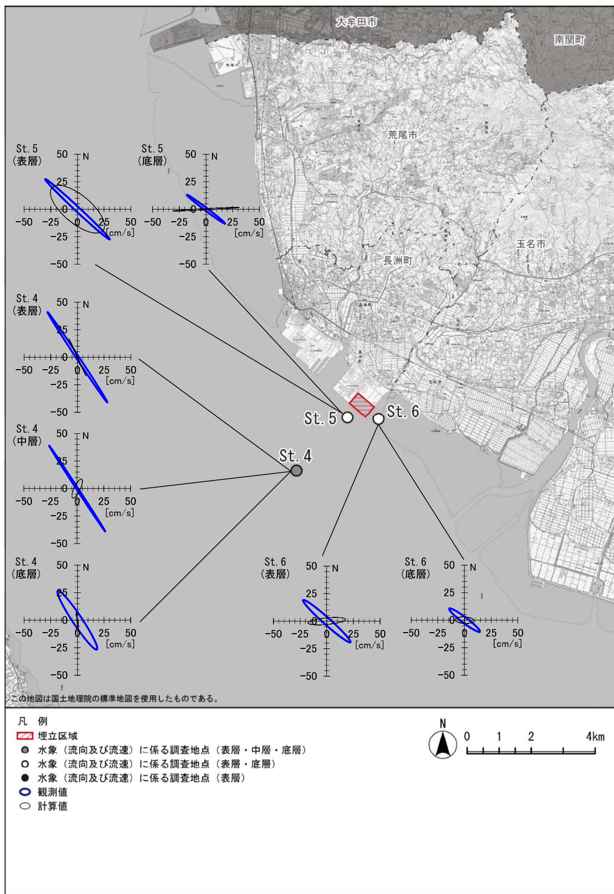
図 7.4-23(1) 調査地点における M_2 分潮の潮流楕円の観測値と計算値との比較（夏季）
