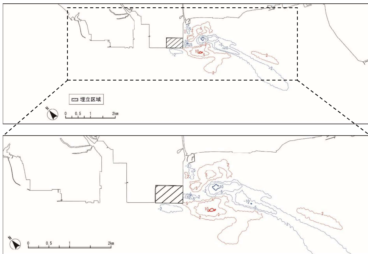
図 7.4-28(3) 流速差図（事業ありー事業なし：夏季下げ潮最強時（ M_2+S_2 分潮））
