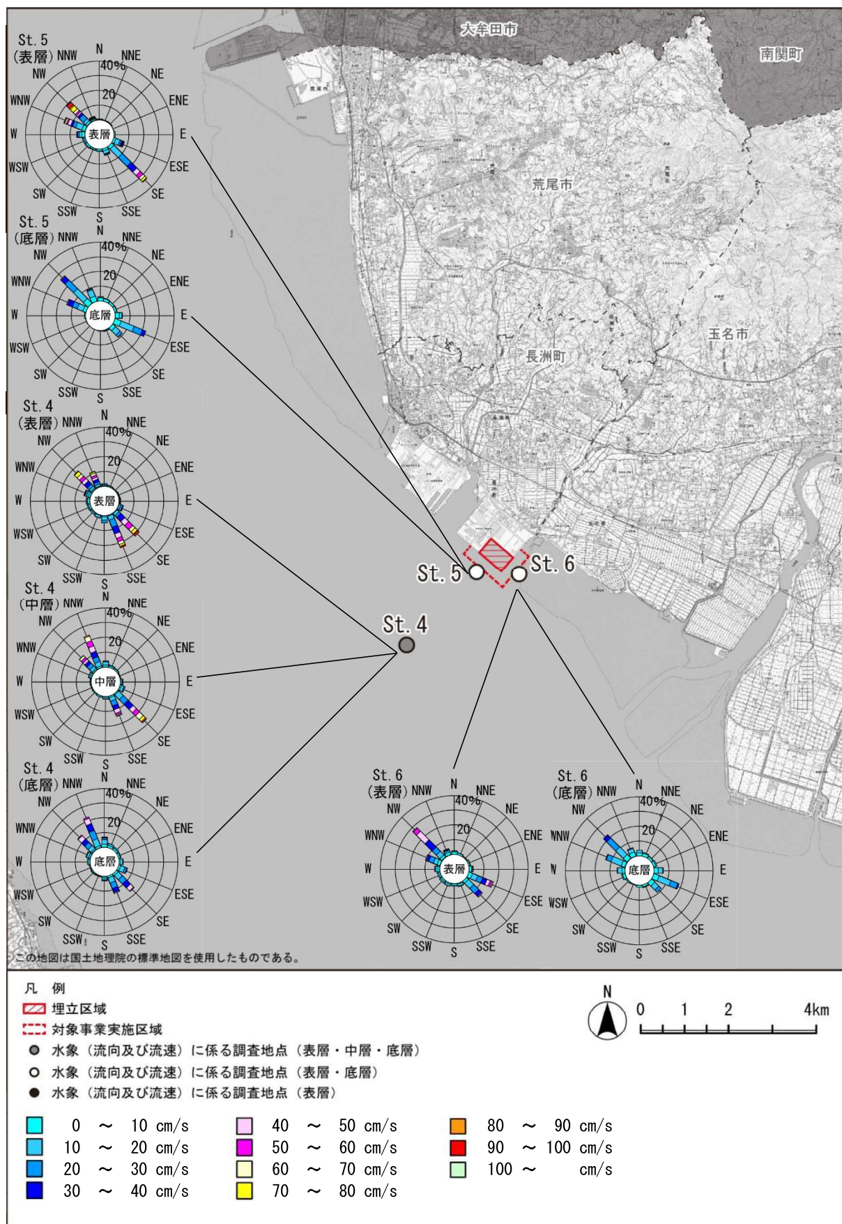
図 7.4-6(1) 流向・流速頻度分布図（夏季）
