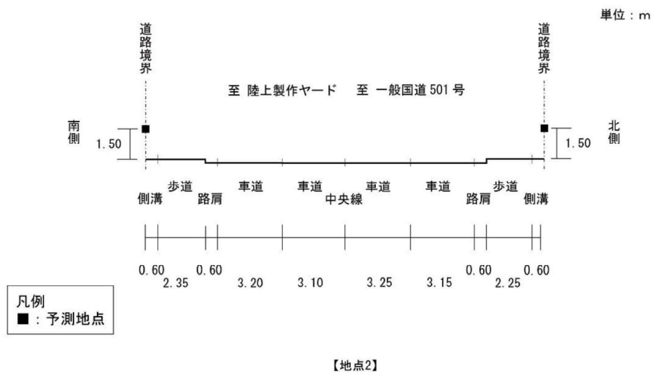
図 7.1-21 予測地点の道路断面構造
