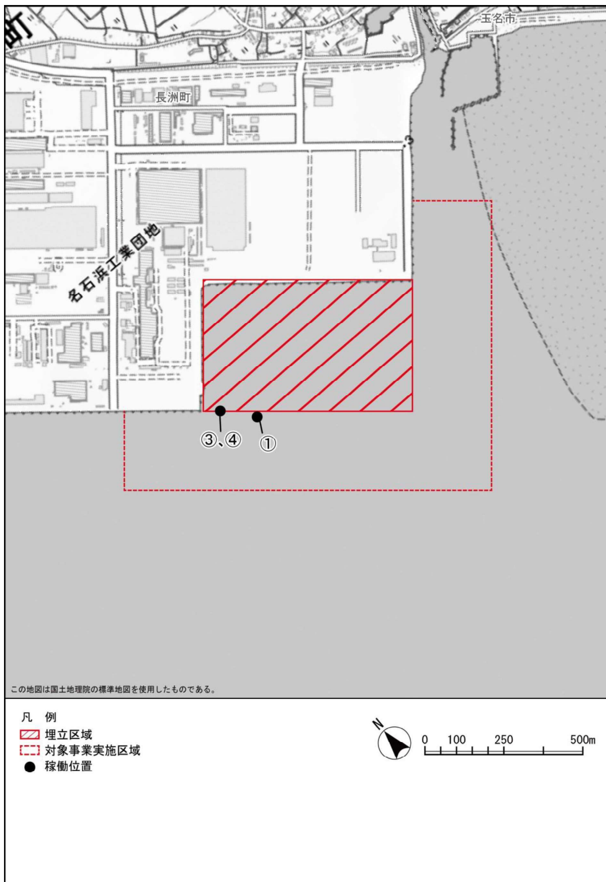
図 7.3-5 建設機械及び工事用船舶の稼働位置
