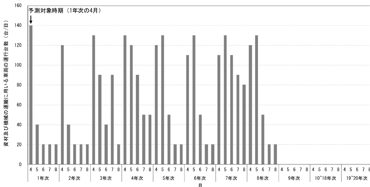
図 7.1-20 (2) 資材及び機械の運搬に用いる車両の日ピーク台数の推移（地点 2）
