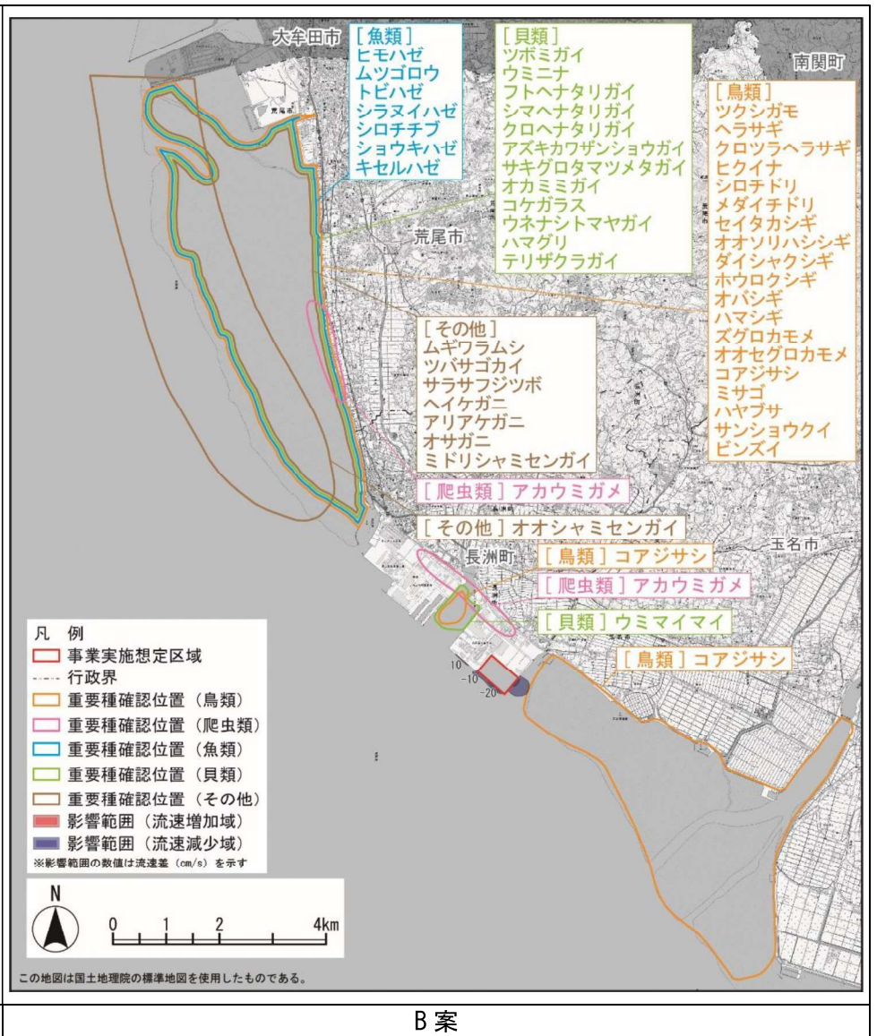
図 4-11(1) 予測結果(上げ潮最強時)
