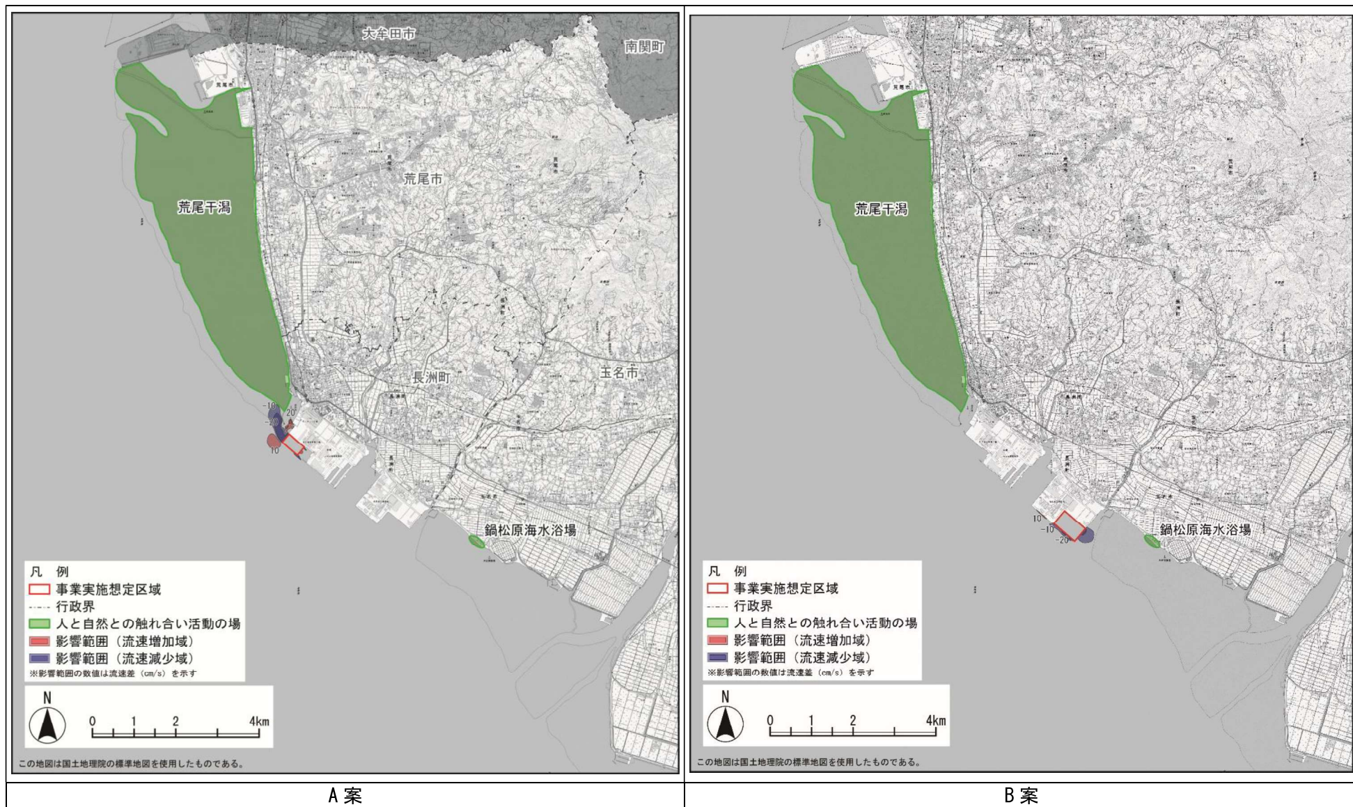
図 4-17(1) 予測結果(上げ潮最強時)
