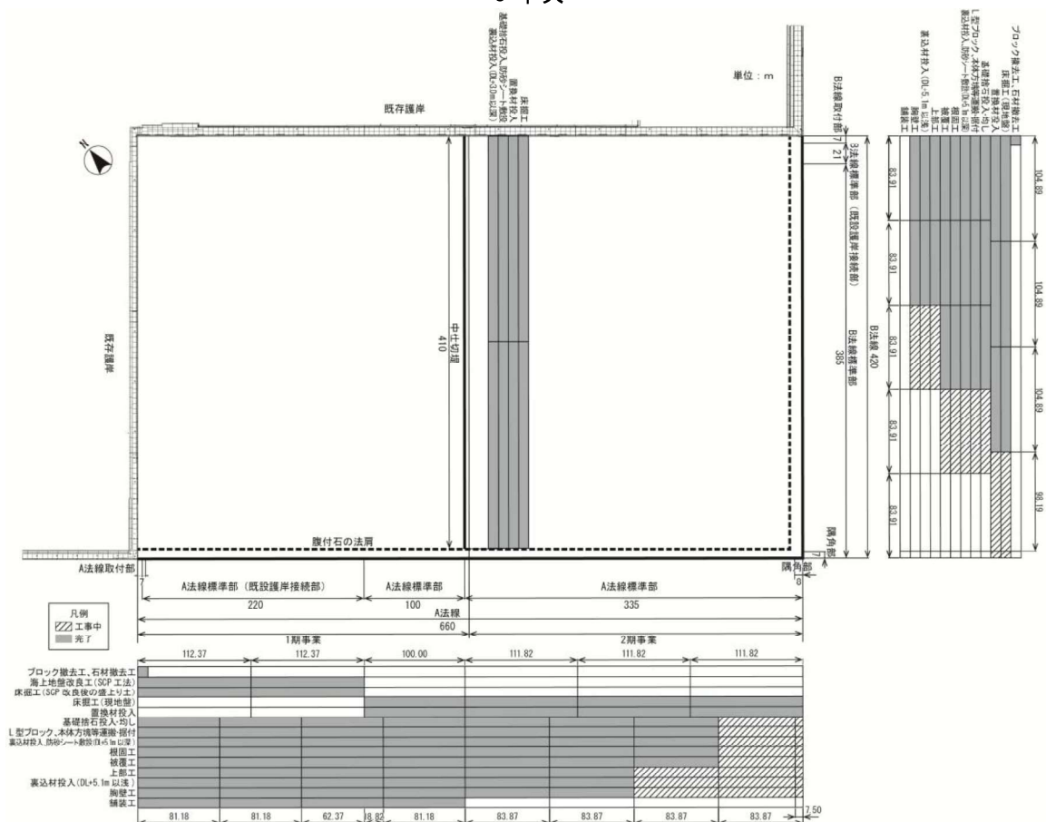
図 2-20 (2) 護岸工の工事進捗図 (2 期)
