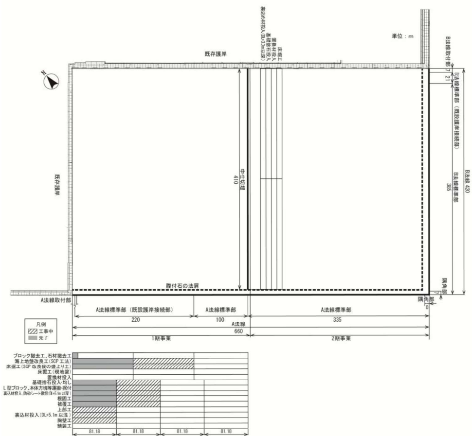
図 2-19(1) 護岸工の工事進捗図 (1 期)
