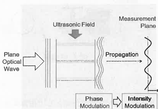
図2 シャドウグラフ法の原理
