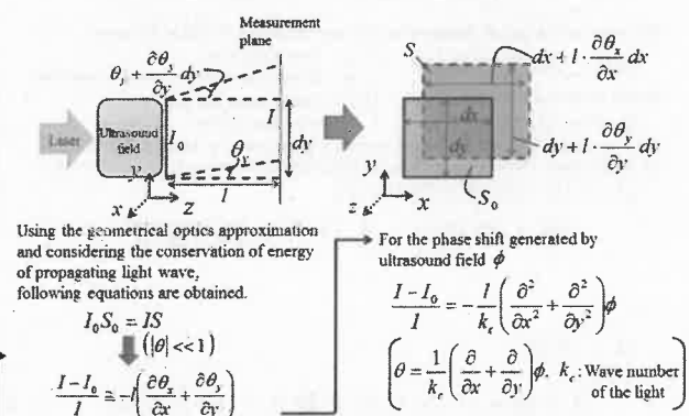
図3 位相変調から振幅変調への変換
