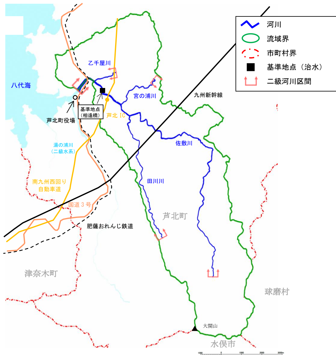
図 3.1 佐敷川水系河川位置図
