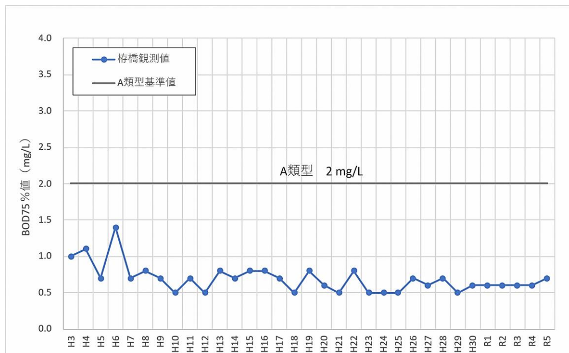
図 2.3 佐敷川榑橋地点 BOD75%値
