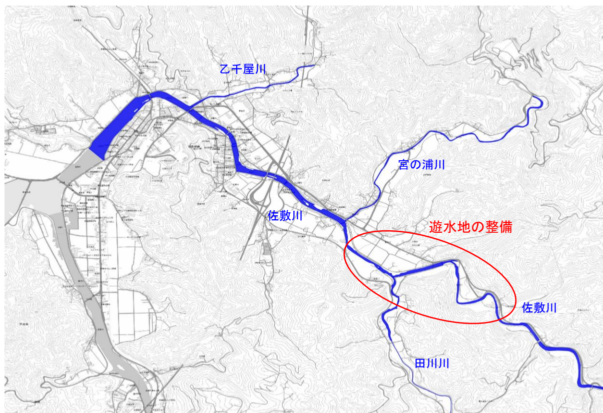
図 5.17 対策の候補地
