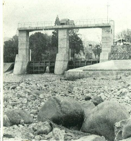
改築成った百太郎溝取水口
