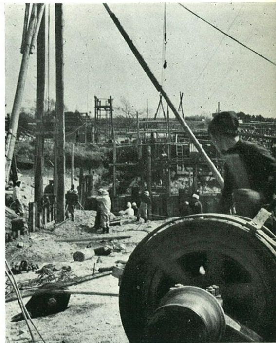
白石堰改築工事現場
