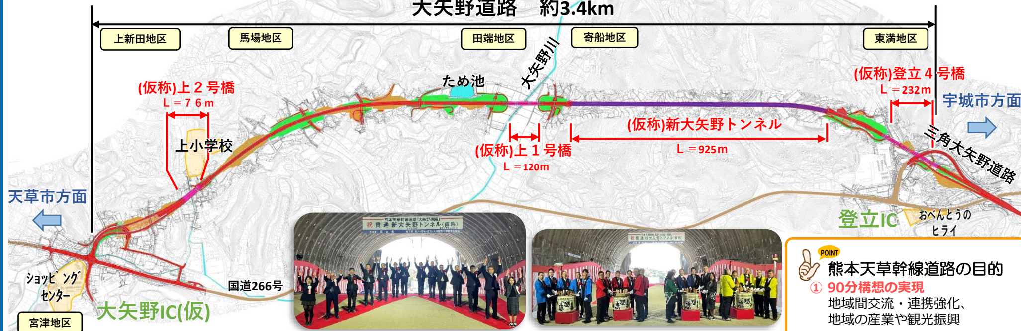
R7.2.24 貫通式の様子
