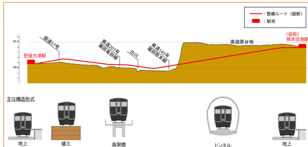
〔鉄道（構造）縦断イメージ〕
