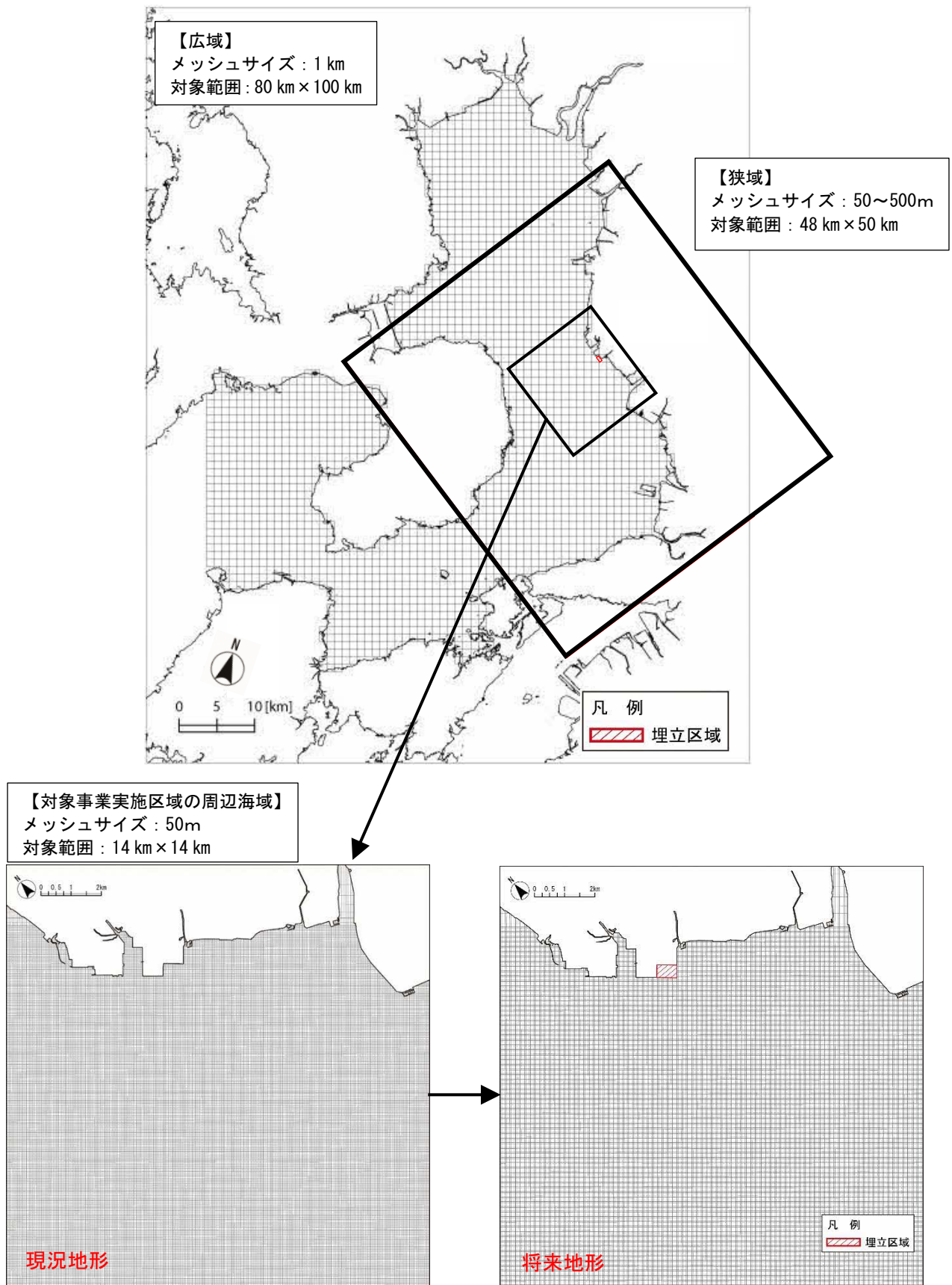
図 7.5-20 格子分割図
