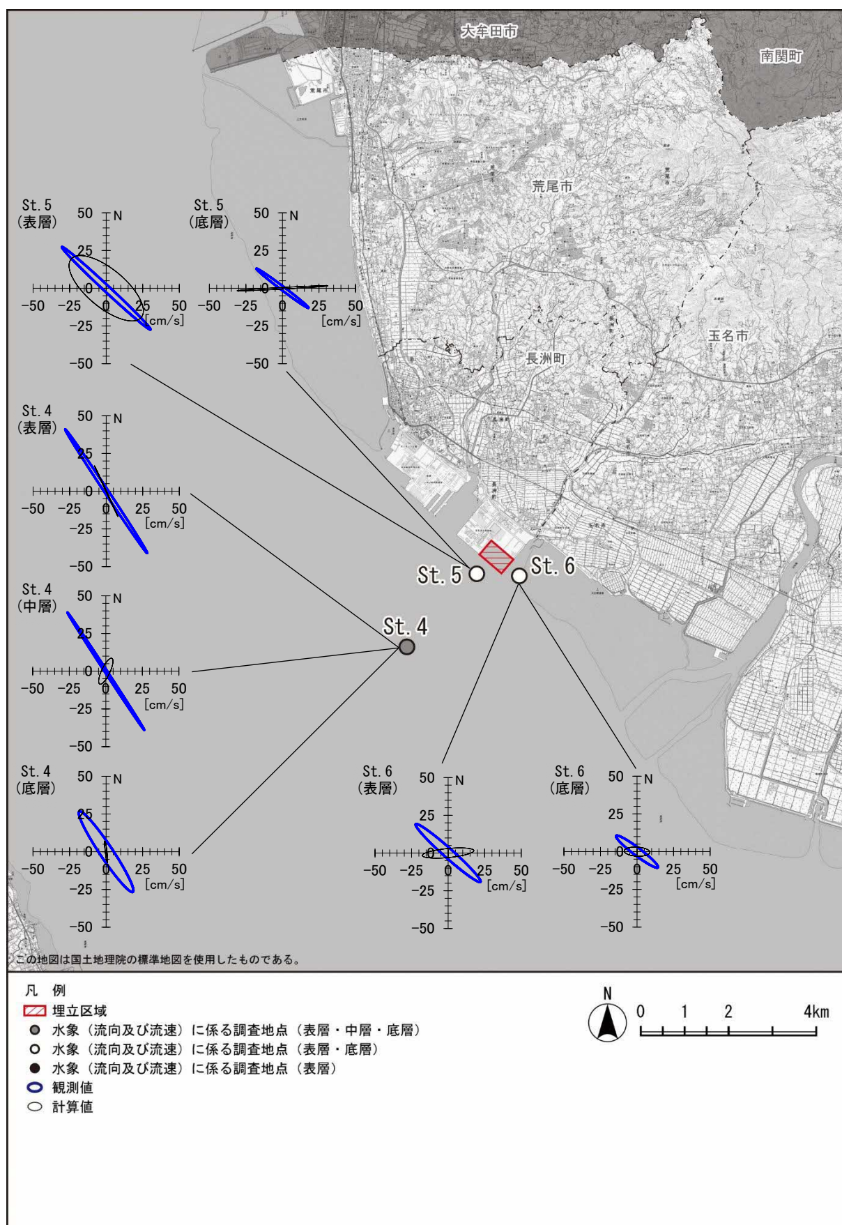
図 7.4-23(1) 調査地点における M_2 分潮の潮流楕円の観測値と計算値との比較（夏季）
