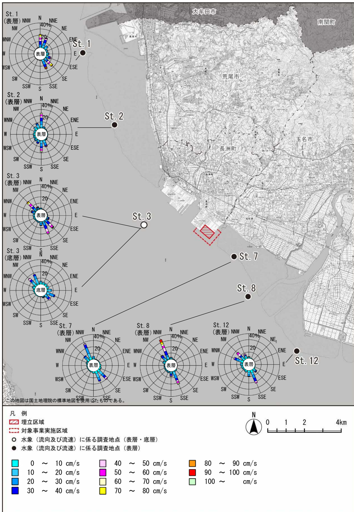
図 7.4-6(2) 流向・流速頻度分布図（夏季）
