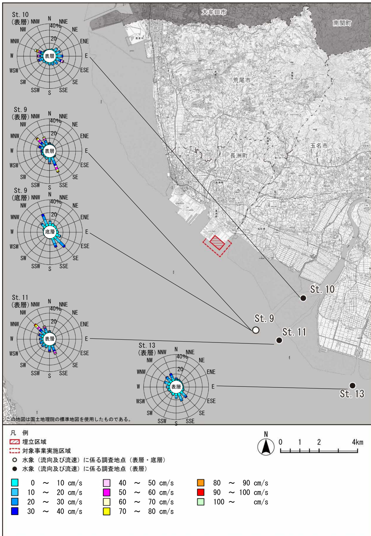
図 7.4-6(3) 流向・流速頻度分布図（夏季）
