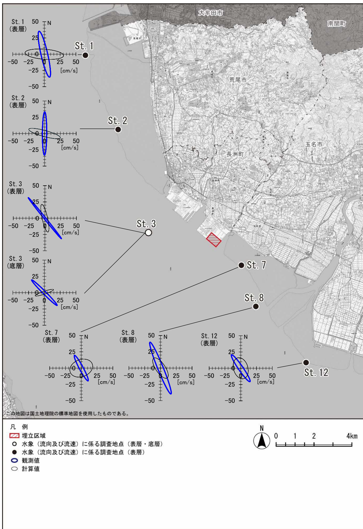
図 7.4-23 (2) 調査地点における M_2 分潮の潮流楕円の観測値と計算値との比較（夏季）
