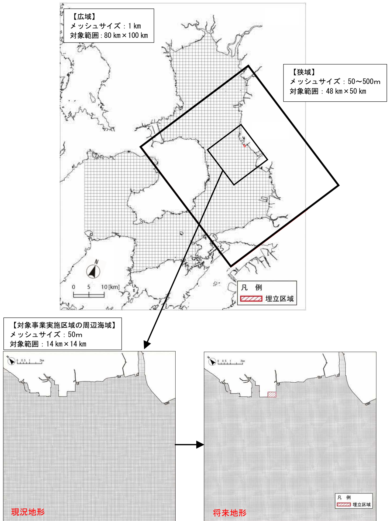
図 7.4-16 格子分割図
