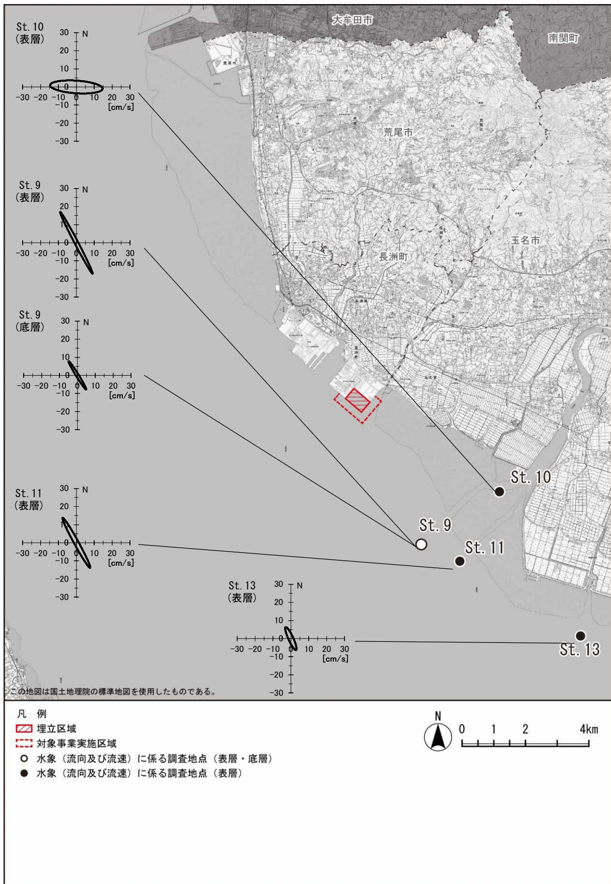
図 7.4-10(3) 潮流楕円図 ( S_2 分潮) (夏季)
