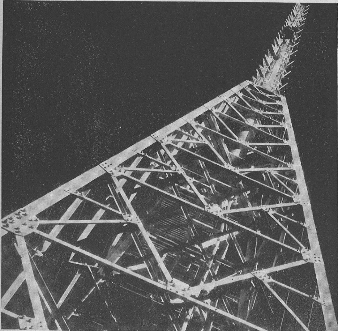
完成ちかし・冬空にメカニツクな美しさをみせるNHK熊本テレビジョン放送局金峰山中継所のテレビ塔
