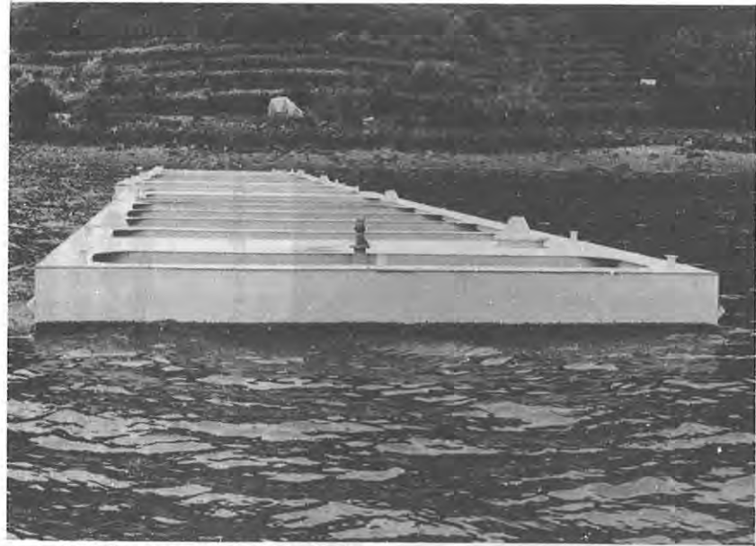
▲御所浦町風口沖に設置された消波堤
