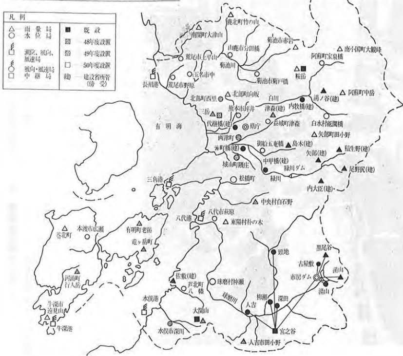
熊本県水防テレメーター設置計画図
