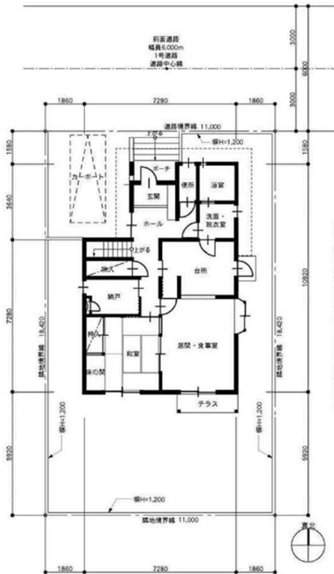
■ 1 階平面図 S=1/150
