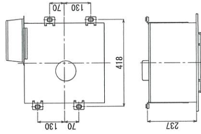
■ 吊下金具DV-4T (別売システム部材) 取付位置(4点吊り)
