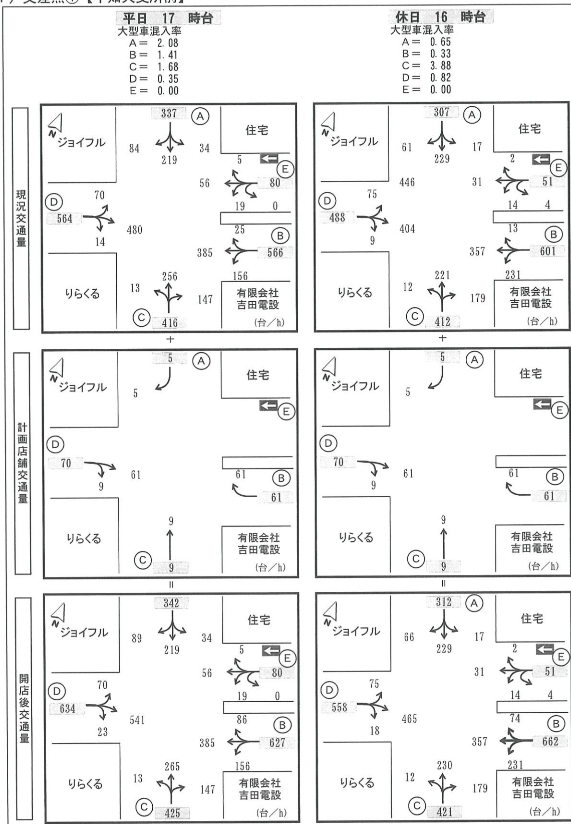
図 5-1 ピーク時交通量 (大型車・小型車計)
