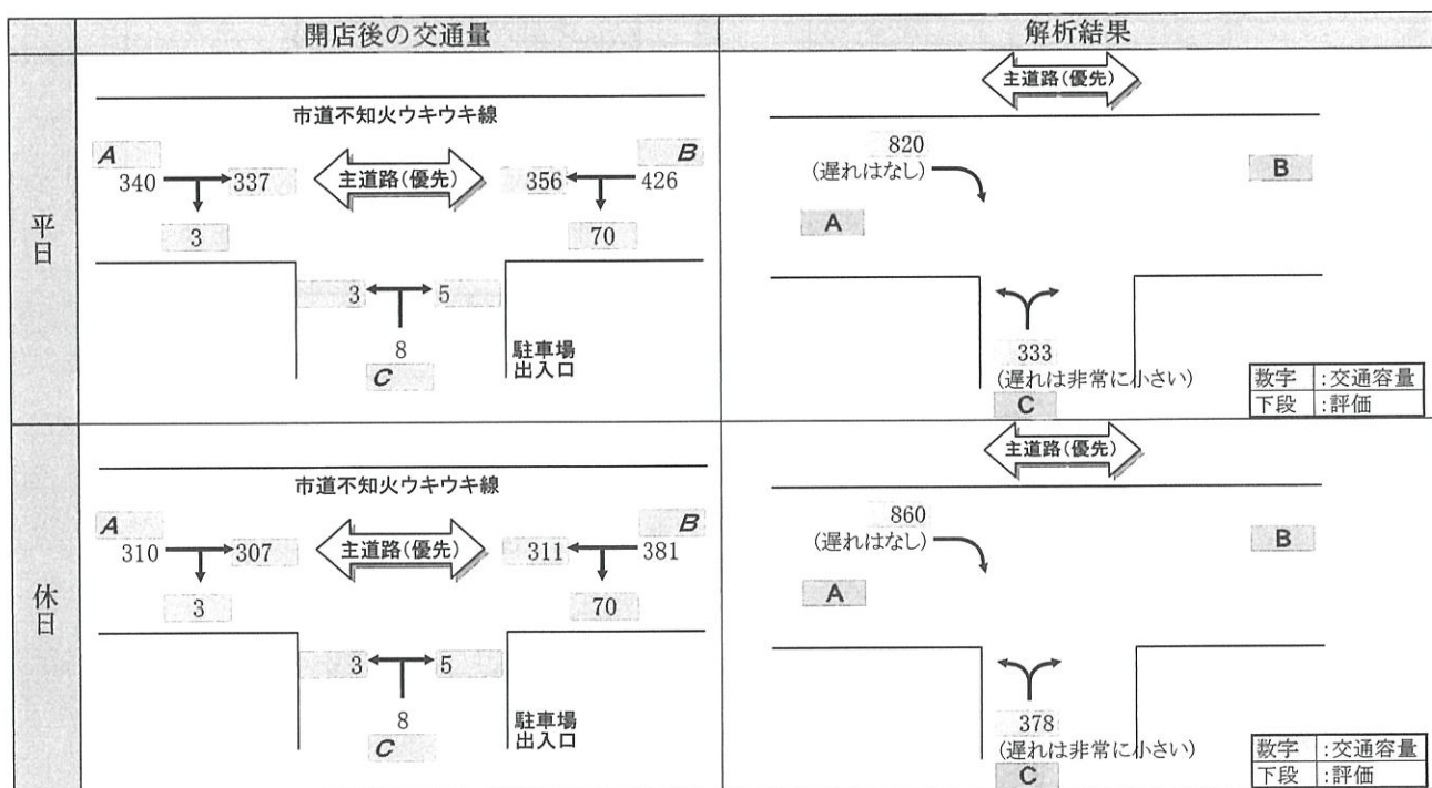
図 5-4 出入口容量計算結果
