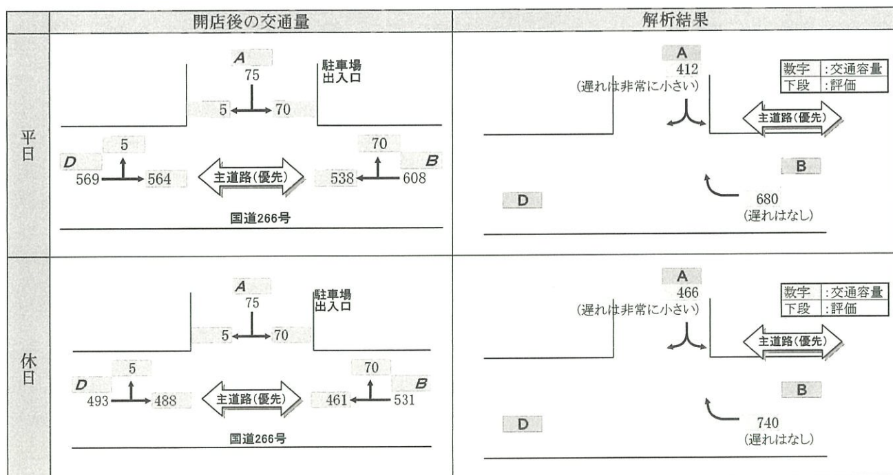
図 5-5 出入口容量計算結果
