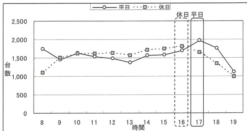
図 2-3 時間帯別断面交通量 (大型車・小型車計)
