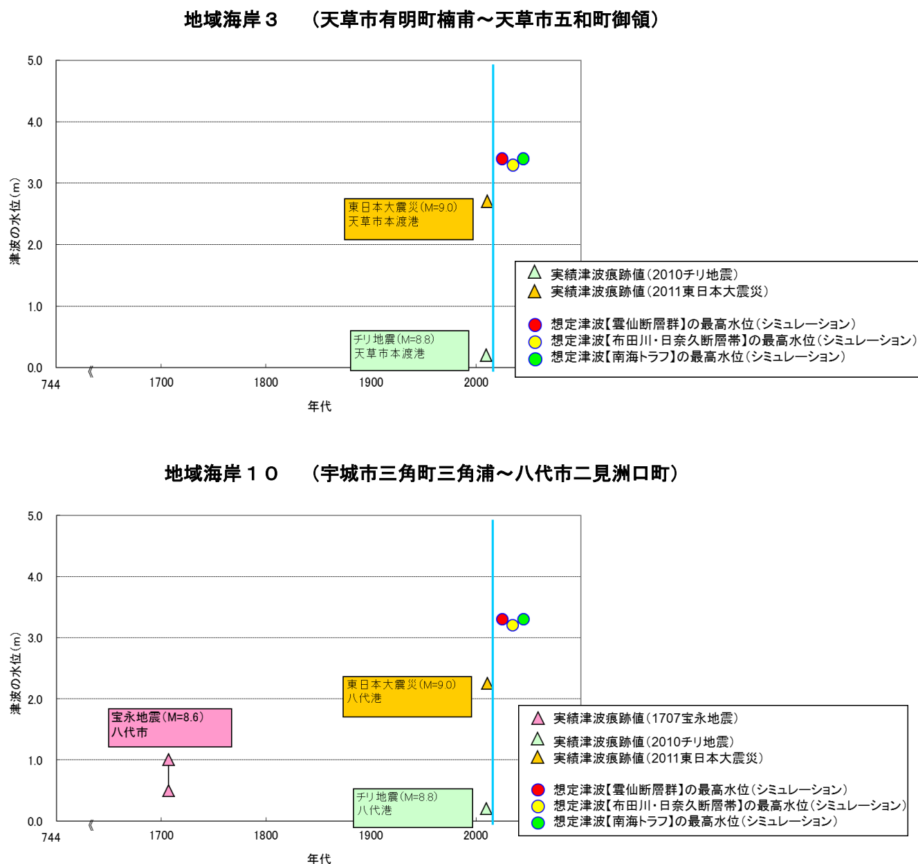
図-4 最大クラスの津波 (L2 津波) の選定例
