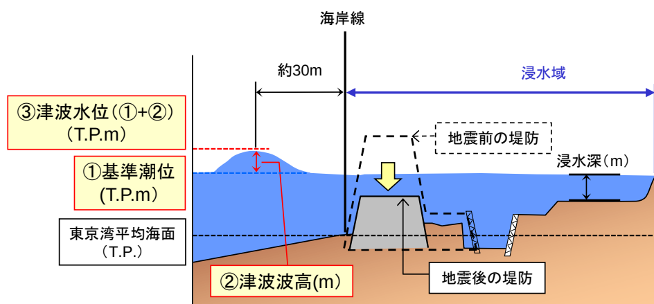
図-2 津波の水位の定義（熊本県）
