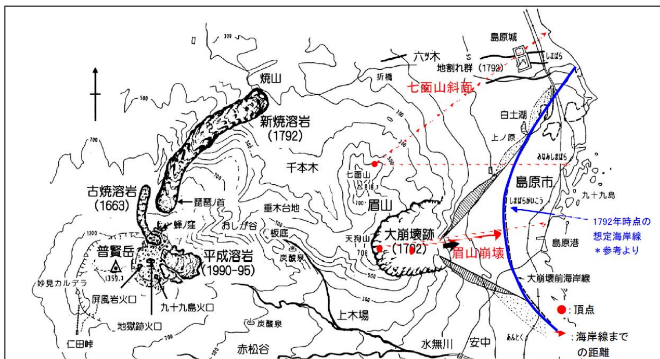
図－5 雲仙岳内の天狗山、七面山、普賢岳の位置図
