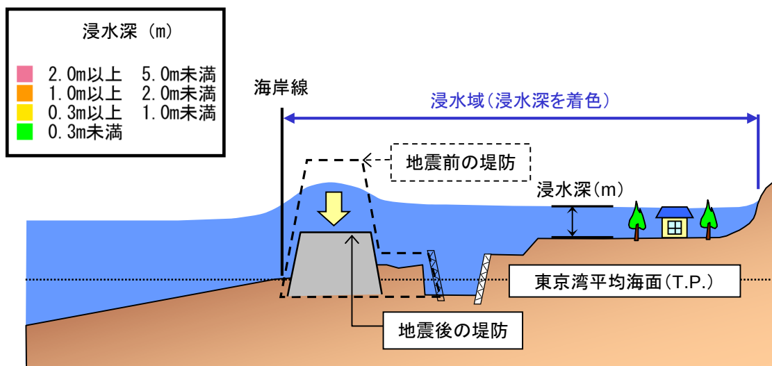
図一2 浸水域と浸水深の模式図
