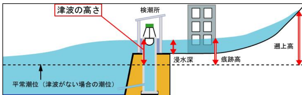
図-1 津波の高さの定義（気象庁）
