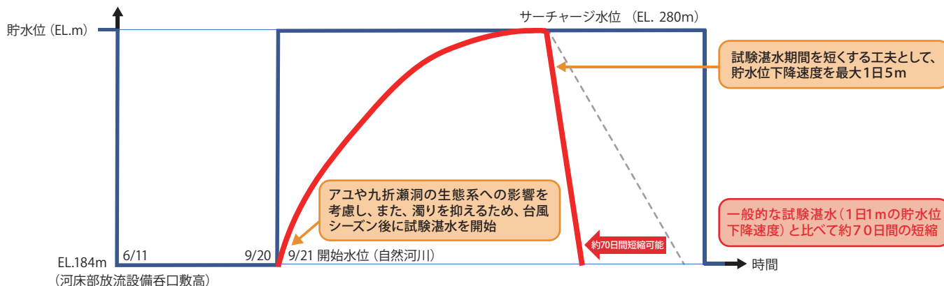
環境影響評価における試験湛水の貯水位イメージ
