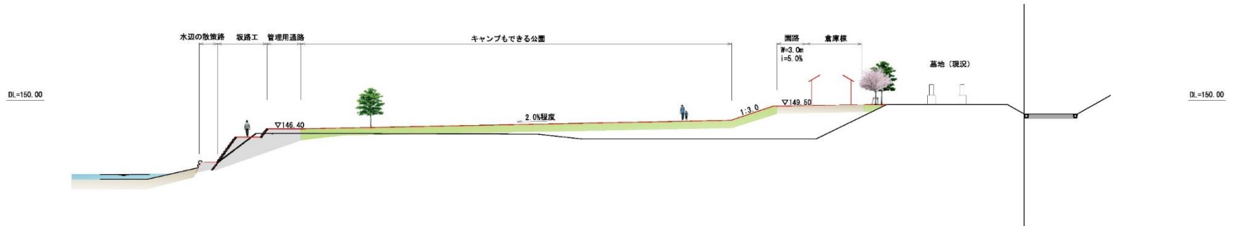
断面-A
