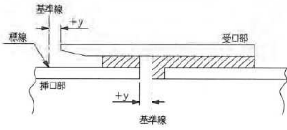
C形
