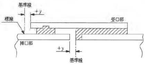
T形
