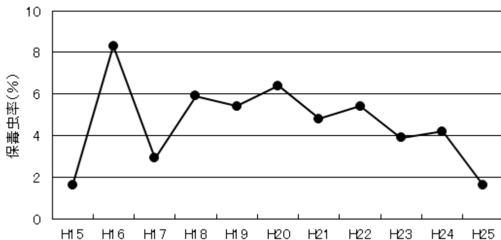
図1 ヒメトビウンカのイネ縞葉枯ウイルス保毒虫率の推移 (H17はネットトラップで捕獲された虫で検定を行った。)
