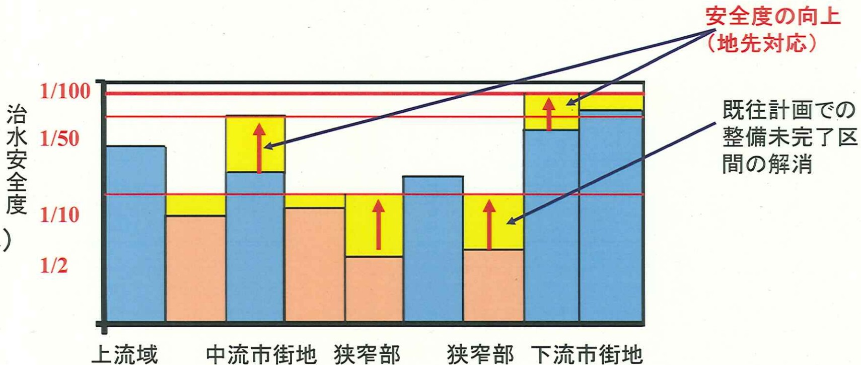
整備計画(上下流方向)イメージ図の案 1
