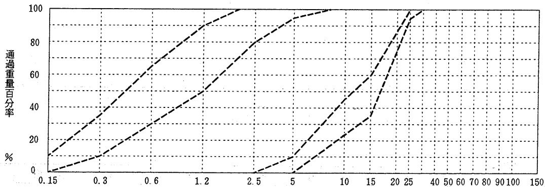
粒度曲線図
