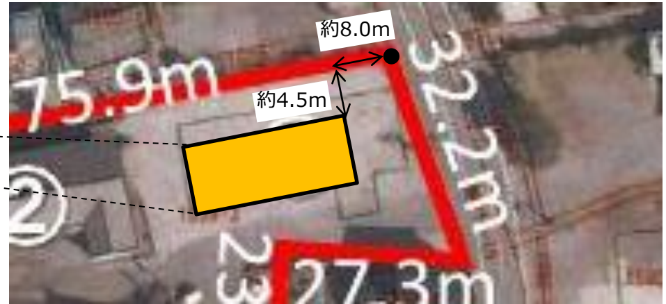
昭和区公民館建設予定地(縦方向×横方向) : 10.45m×18.05m
