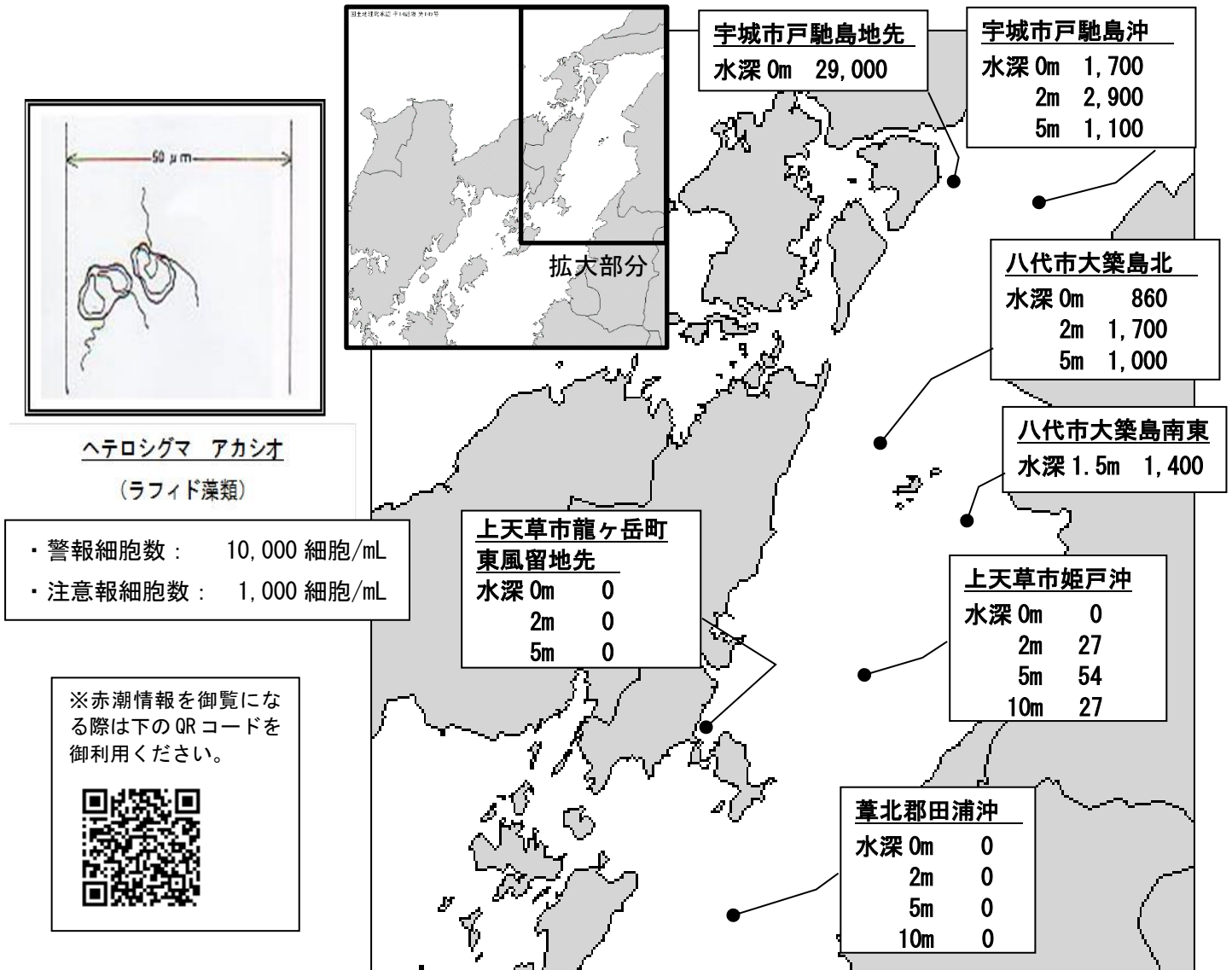
図 海水1mLあたりのヘテロシグマ アカシオの細胞数
