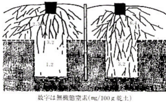
図2 堆肥の施用位置とトマトの根群分布 数字は無機態窒素(mg/100g 乾土)
