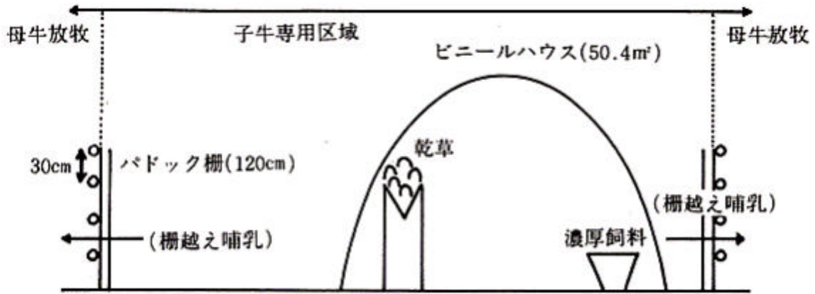
図1 親子分離放牧施設概要（柵越え哺乳）
